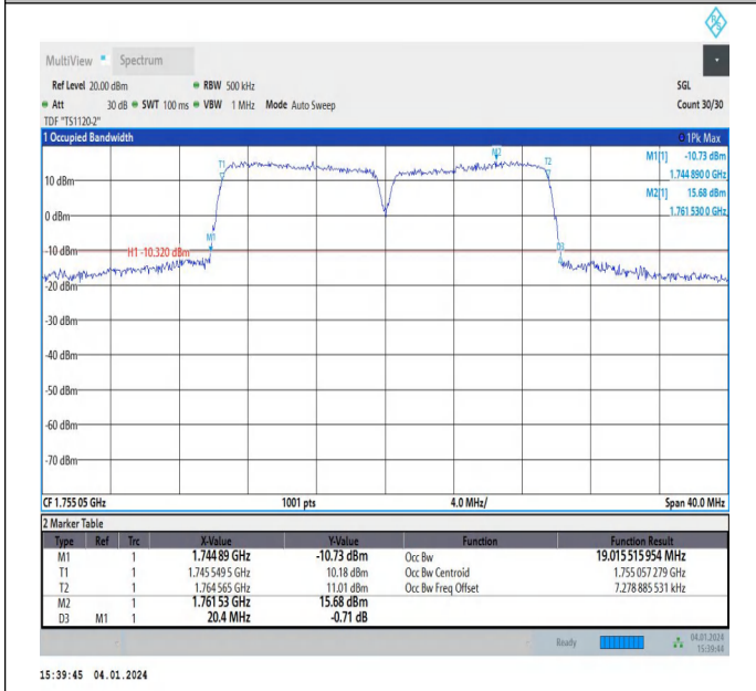
66-66-10MHz-10MHz-64QAM-64QAM-132373-132472-50RB#0-50RB#0-PASS
