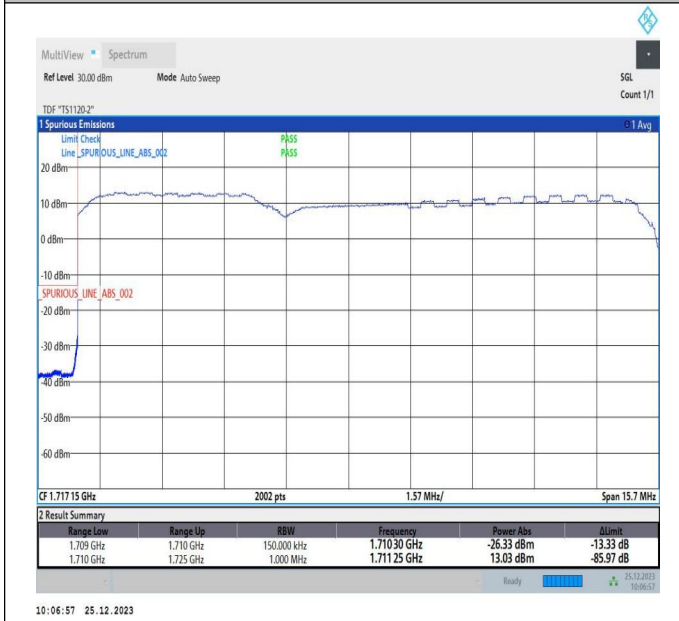
5MHz-10MHz_QPSK@QPSK-QPSK@QPSK_132000-132072_2_25RB#0@25RB#0-50RB#0@50RB#0
