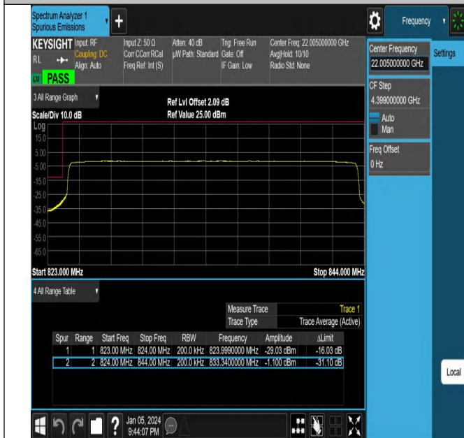
NTNV_N5_PC3_15_20_L_TID16_#1
