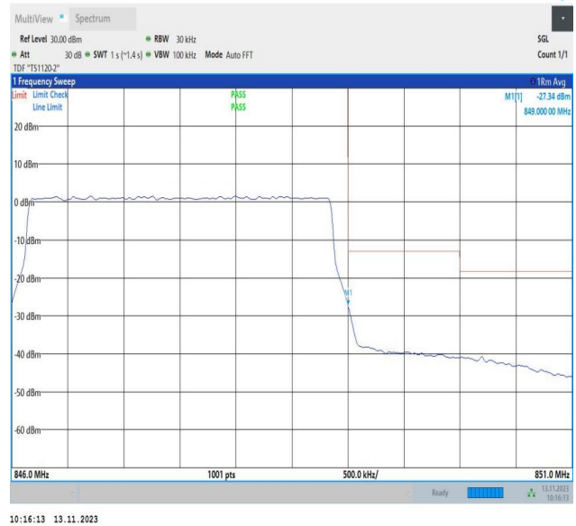
Band5_3MHz_16QAM_20635_15RB#0
