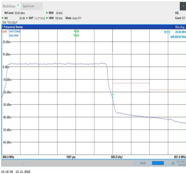
Band5_3MHz_QPSK_20635_15RB#0
