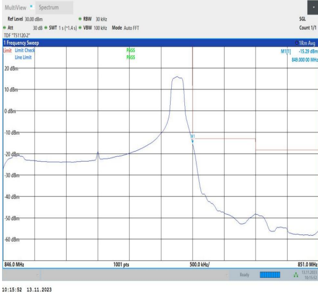
Band5_3MHz_QPSK_20635_1RB#14
