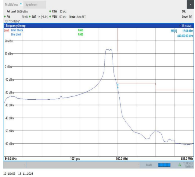
Band5_3MHz_16QAM_20635_1RB#14
