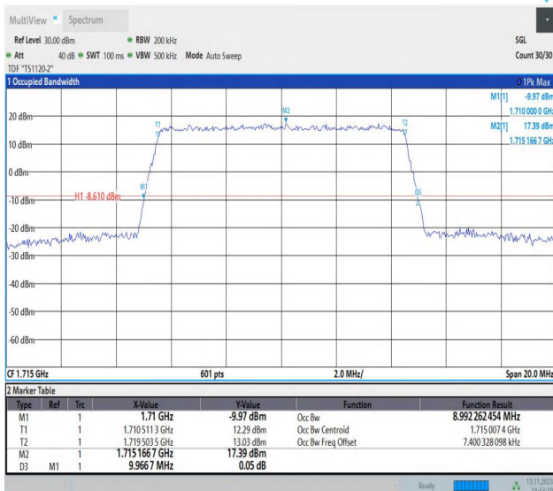
Band4-10MHz-QPSK-20000-50RB#0-PASS
