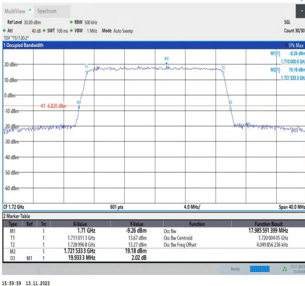
Band4-20MHz-QPSK-20050-100RB#0-PASS
