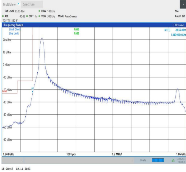
Band2_10MHz_QPSK_18650_1RB#0
