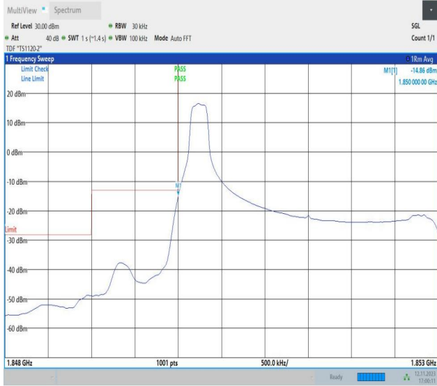
Band2_3MHz_QPSK_18615_1RB#0
