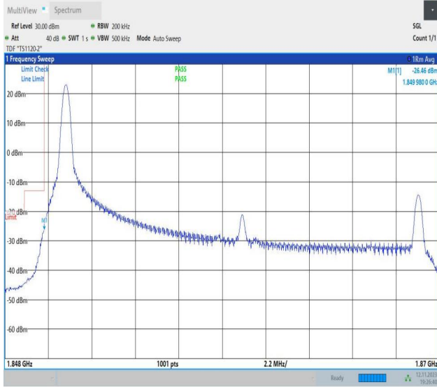
Band2_20MHz_QPSK_18700_1RB#0
