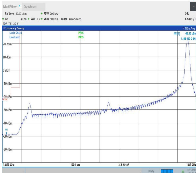
Band2_20MHz_QPSK_18700_1RB#99
