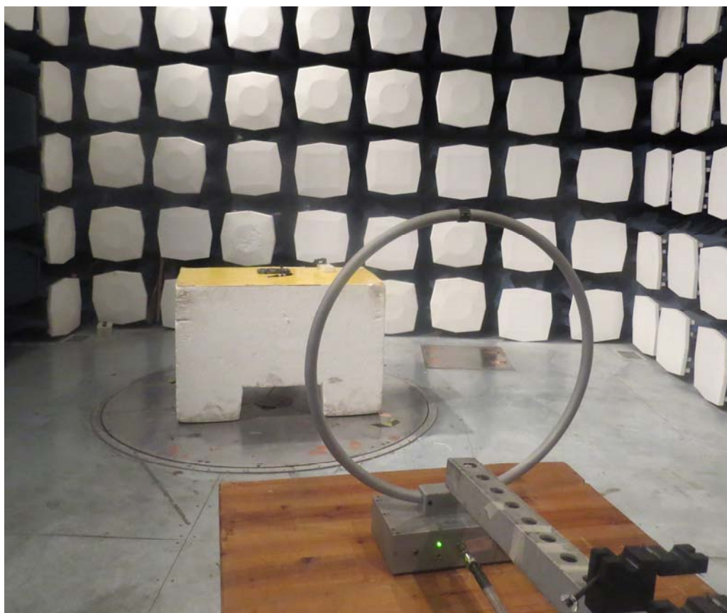
9kHz-30MHz
