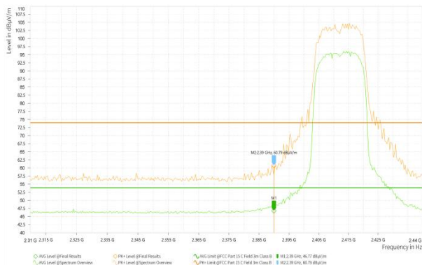
802.11n 20M_2412_edge
