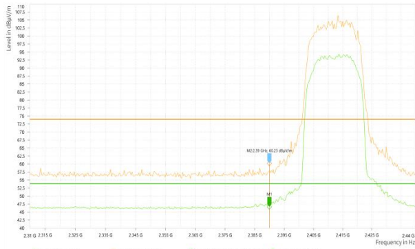
802.11ax 20M_2412_edge
