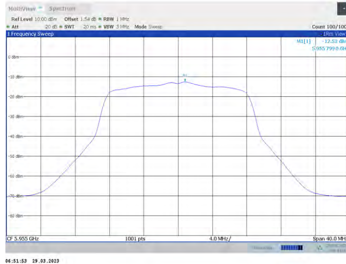
11a-CDD_Ant1_5955
