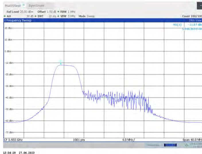
11ax20MIMO_Ant0_5955_52Tone_RU37
