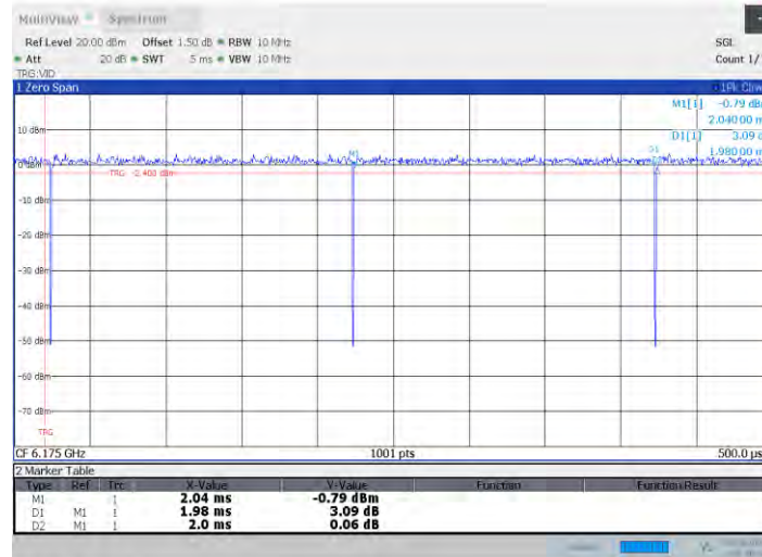
11a-CDD_Ant1_6175
