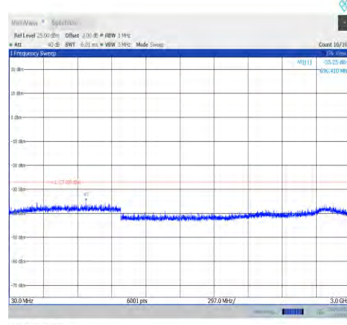
11a-CDD-Ant1-6415-30~3000-PASS
