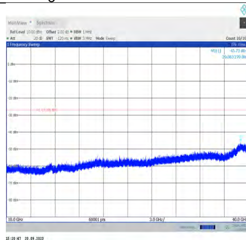
11a-CDD-Ant1-6415-10000~40000-PASS
