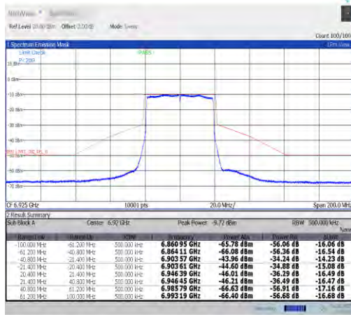
NTVN-11ax40MIMO-Ant0-6925-PASS
