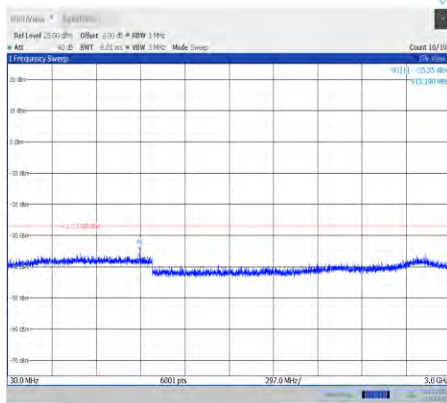
11ax40MIMO-Ant0-6925-30~3000-PASS
