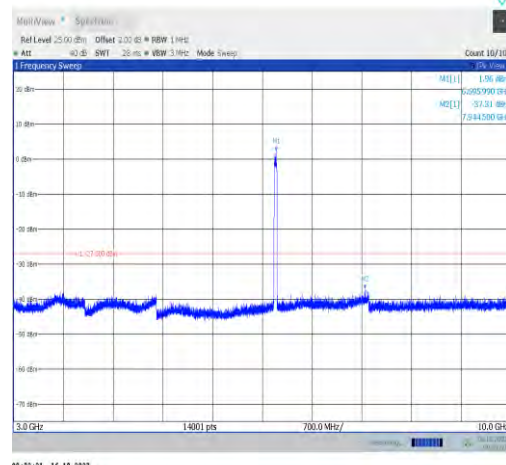
11ax40MIMO-Ant0-6685-3000~10000-PASS
