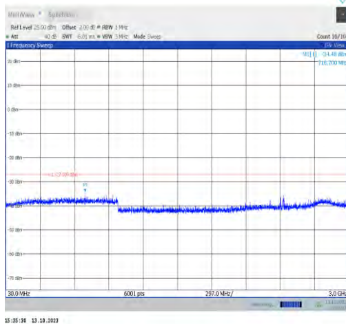
11ax20MIMO-Ant0-6695-30~3000-PASS
