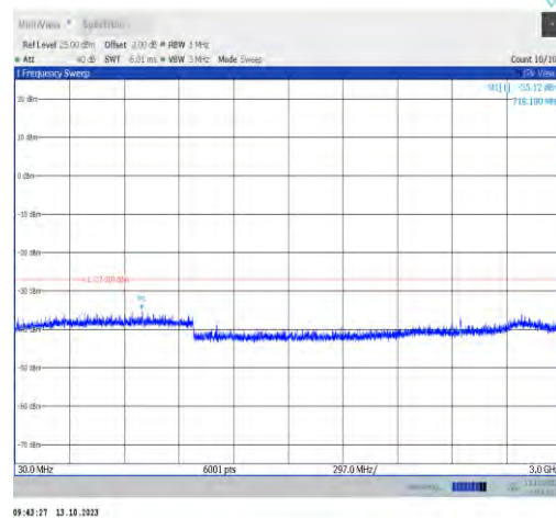
11a-CDD-Ant1-6535-30~3000-PASS
