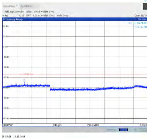
11ax40MIMO-Ant0-6445-30~3000-PASS
