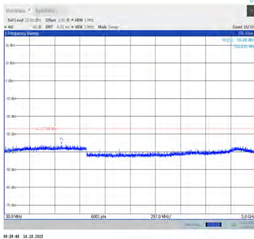
11ax40MIMO-Ant0-6885-30~3000-PASS
