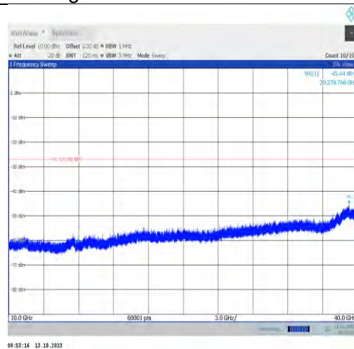
11a-CDD-Ant1-6695-10000~40000-PASS
