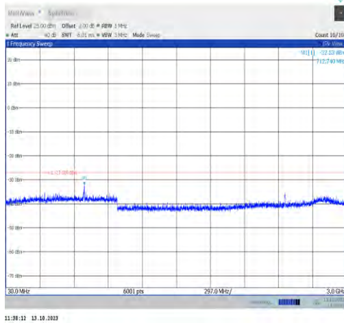
11a-CDD-Ant0-7115-30~3000-PASS
