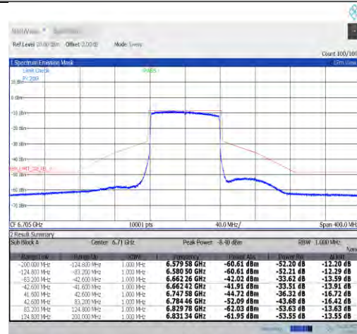
NTVN-11ax80MIMO-Ant1-6705-PASS
