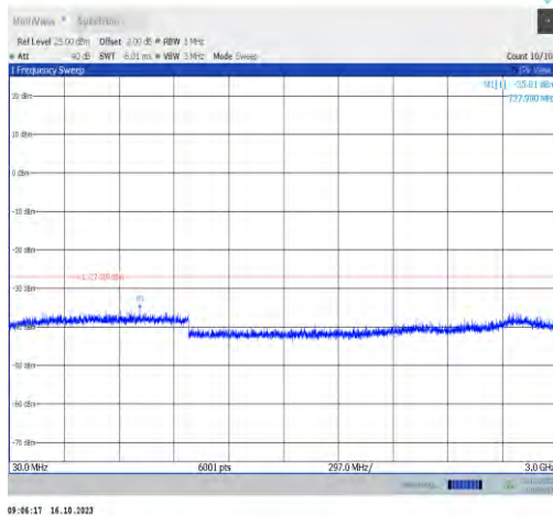
11ax40MIMO-Ant0-6485-30~3000-PASS
