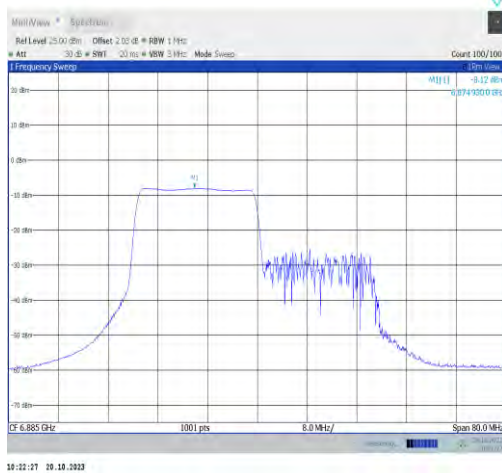
11ax40MIMO-Ant0-6885-PASS
