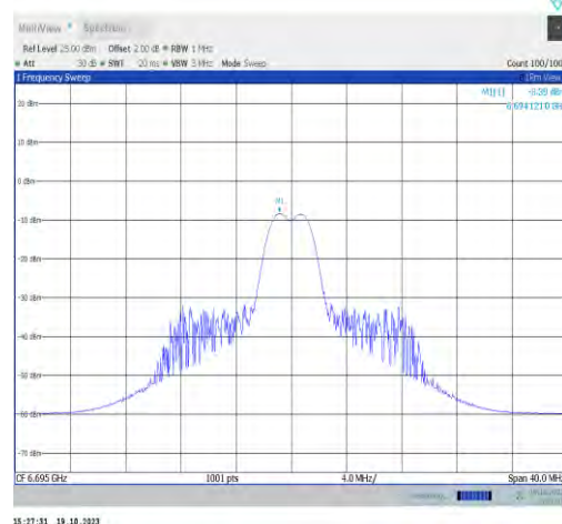
11ax20MIMO-Ant1-6695-PASS
