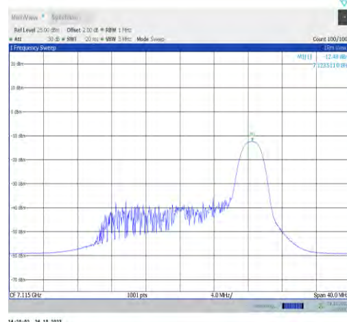
11ax20MIMO-Ant1-7115-PASS
