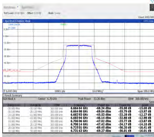
NTNV-11a-CDD-Ant0-6695-PASS
