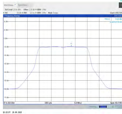
11a-CDD-Ant1-6435-PASS
