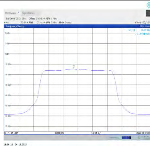
11ax20MIMO-Ant1-7115-PASS
