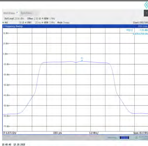
11ax20MIMO-Ant0-6875-PASS
