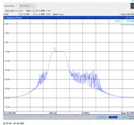
11ax20MIMO-Ant0-6995-PASS
