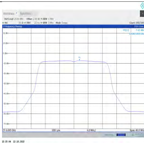
11ax20MIMO-Ant0-6695-PASS
