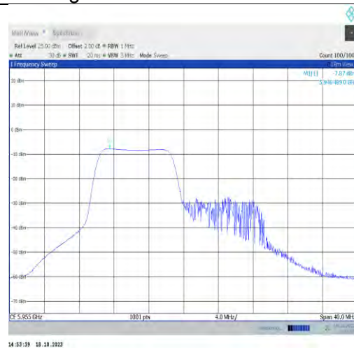
11ax20MIMO-Ant1-5955-PASS
