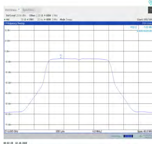
11a-CDD-Ant1-6695-PASS
