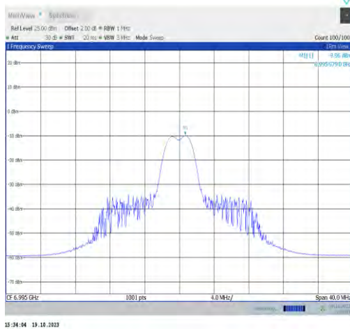
11ax20MIMO-Ant0-6995-PASS
