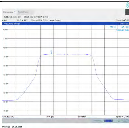
11a-CDD-Ant0-6855-PASS
