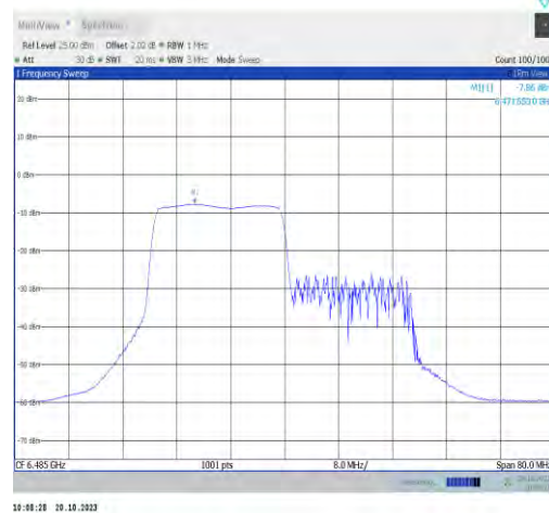
11ax40MIMO-Ant1-6485-PASS
