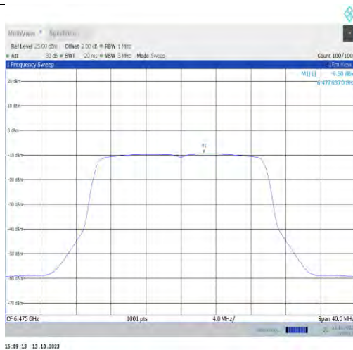
11ax20MIMO-Ant0-6475-PASS
