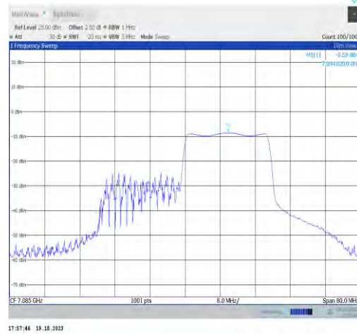
11ax40MIMO-Ant1-7085-PASS
