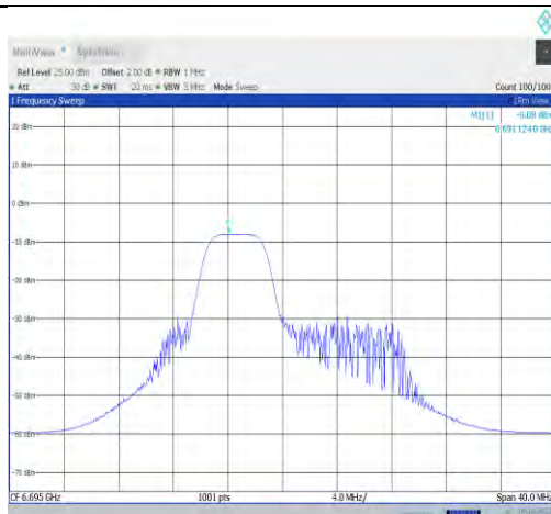
11ax20MIMO-Ant1-6695-PASS
