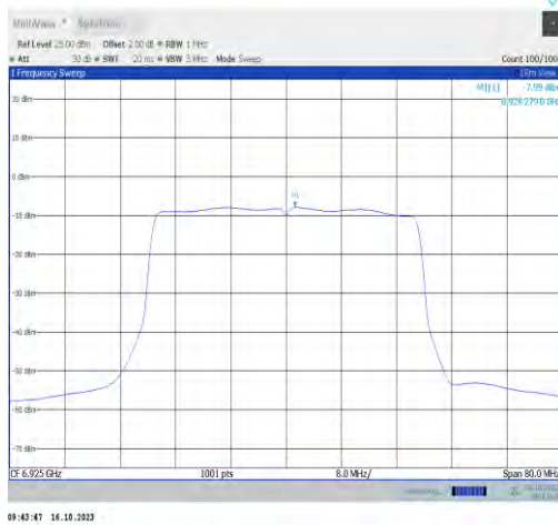
11ax40MIMO-Ant0-6925-PASS
