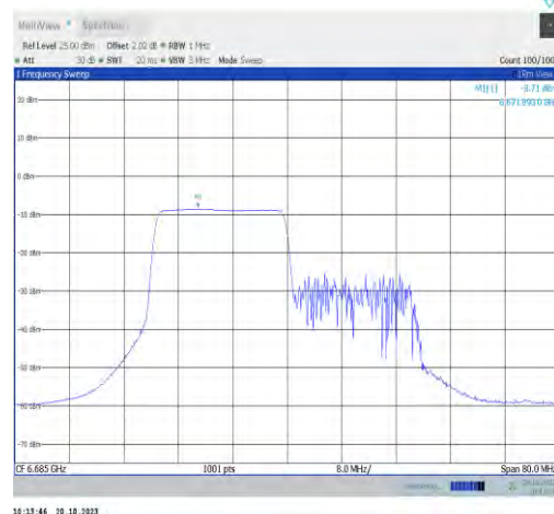
11ax40MIMO-Ant1-6685-PASS
