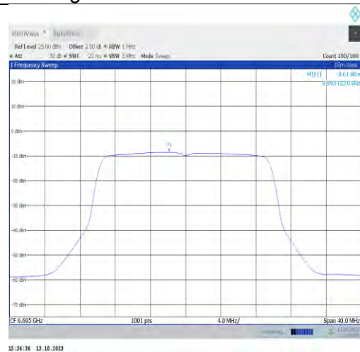
11ax20MIMO-Ant1-6695-PASS
