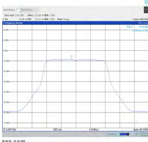
11a-CDD-Ant0-6695-PASS
