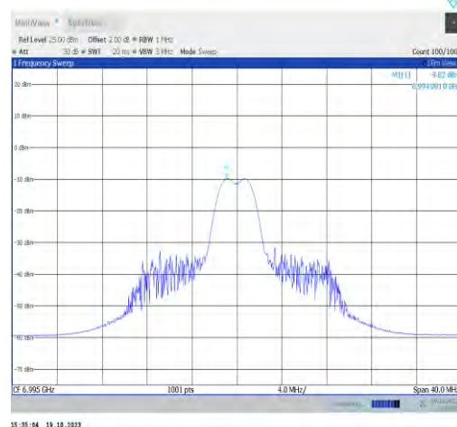
11ax20MIMO-Ant1-6995-PASS
