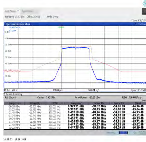
NTVN-11ax20MIMO-Ant1-6415-PASS
