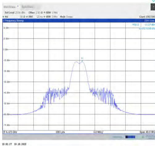
11ax20MIMO-Ant0-6475-PASS
