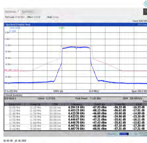
NTVN-11ax20MIMO-Ant1-6435-PASS
