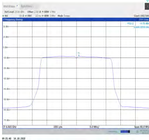
11ax40MIMO-Ant0-6685-PASS
