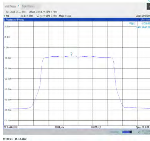
11ax40MIMO-Ant1-6485-PASS
