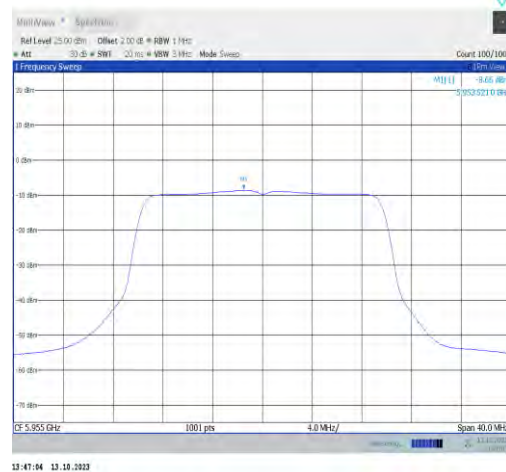
11ax20MIMO-Ant1-5955-PASS
