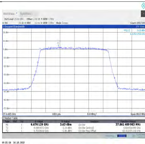
11ax40MIMO-Ant0-6685-PASS
