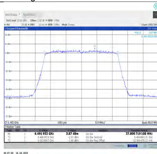
11ax40MIMO-Ant1-6485-PASS
