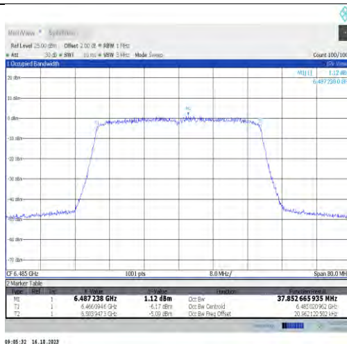
11ax40MIMO-Ant0-6485-PASS
