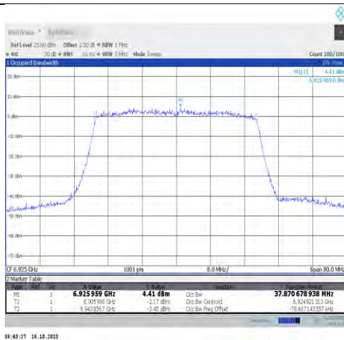
11ax40MIMO-Ant0-6925-PASS
