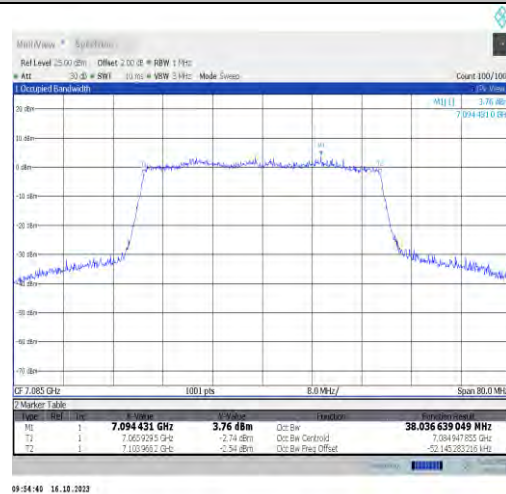
11ax40MIMO-Ant1-7085-PASS
