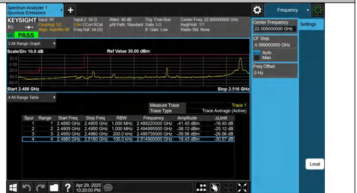
Band41-20MHz-QPSK-39750-1RB#99-PASS
