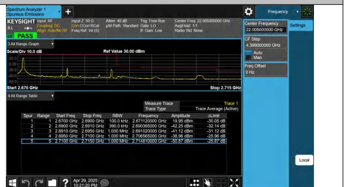
Band41-20MHz-QPSK-41490-1RB#0-PASS
