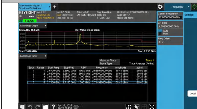
Band41-20MHz-QPSK-41490-1RB#99-PASS
