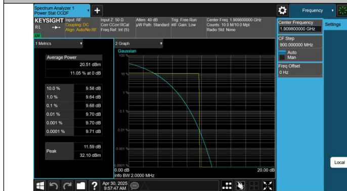
GSM1900-810-0-PASS
