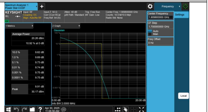
GPRS1900-810-0-PASS
