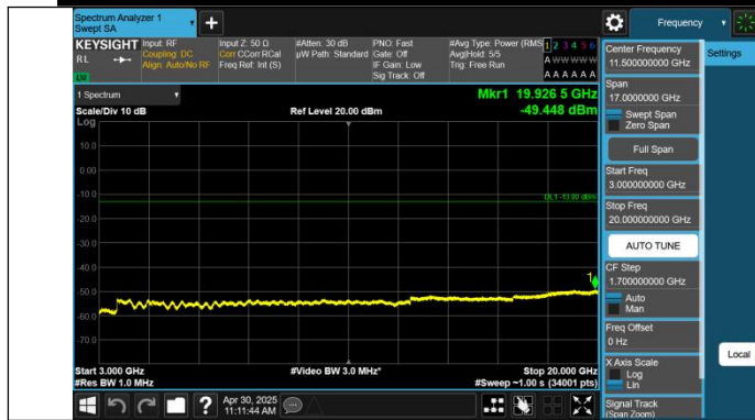
GPRS1900-661-0-3000~20000MHz-PASS
