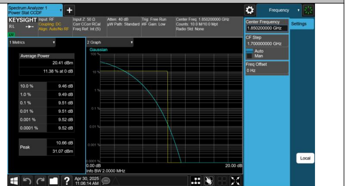
GPRS1900-512-0-PASS
