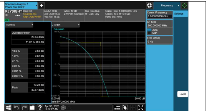
GSM1900-661-0-PASS
