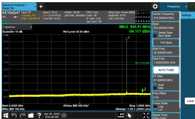
GSM850-128-5-30~1000MHz-PASS
