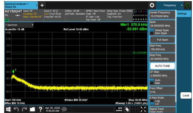
GSM850-128-5-0.15~30MHz-PASS
