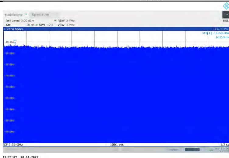
Master—11ac80SISO 5530
