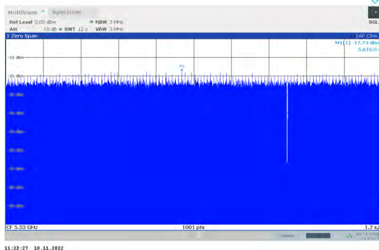
Master—11ac80SISO 5530
