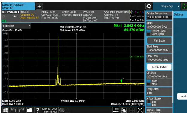
Band66-20MHz-QPSK-132072-1RB#99-1000~3000-PASS
