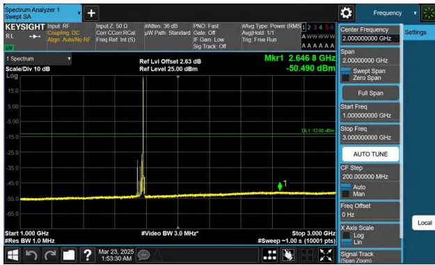
Band66-20MHz-QPSK-132572-1RB#99-1000~3000-PASS
