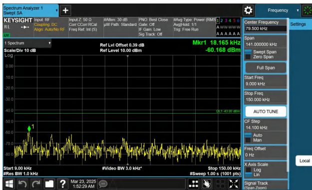
Band66-20MHz-QPSK-132572-1RB#0-0.009~0.15-PASS
