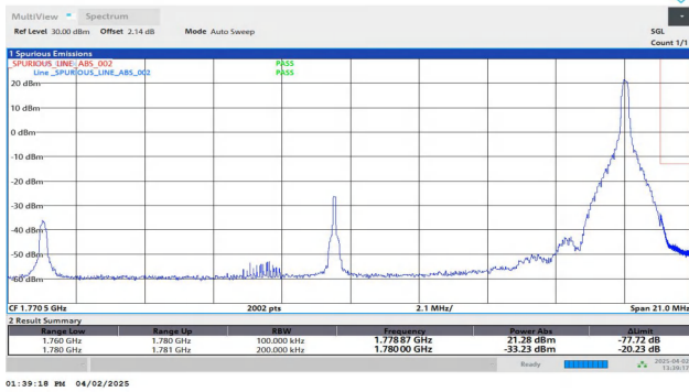
Band66-20MHz-QPSK-132572-1RB#99-PASS
