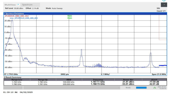
Band66-20MHz-QPSK-132572-1RB#0-PASS
