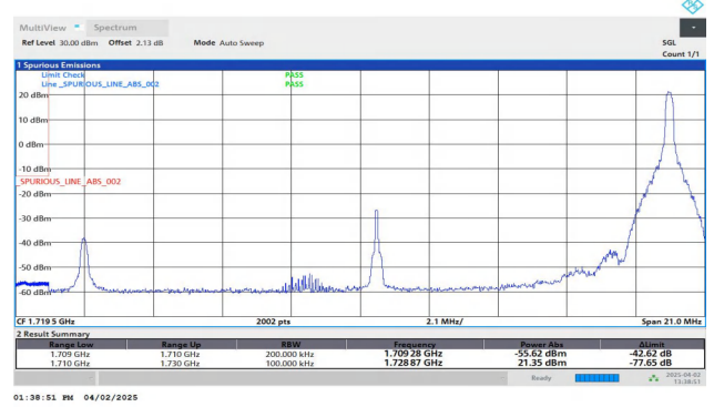
Band66-20MHz-QPSK-132072-1RB#99-PASS
