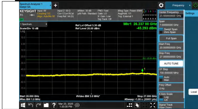
Band41-10MHz-QPSK-41540-1RB#0-20000-PASS
