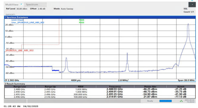
Band41-20MHz-QPSK-39750-1RB#99-PASS
