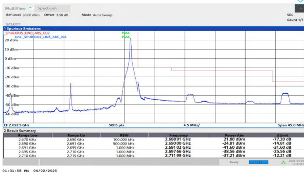
Band41-20MHz-QPSK-41490-1RB#99-PASS
