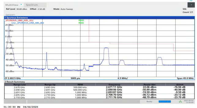
Band41-20MHz-QPSK-41490-1RB#0-PASS
