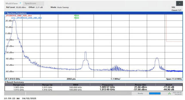
Band25-10MHz-QPSK-26640-1RB#0-PASS
