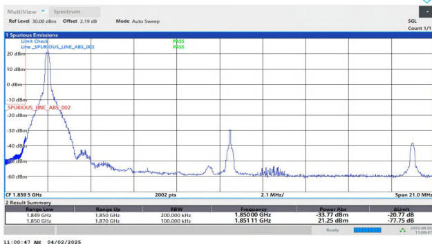
Band25-20MHz-QPSK-26140-1RB#0-PASS
