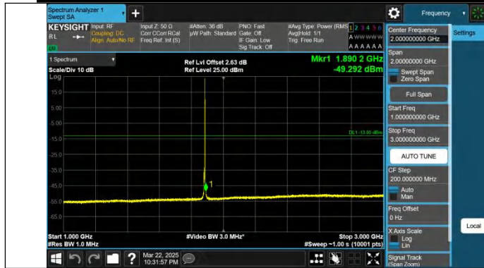
Band25-3MHz-QPSK-26365-1RB#14-1000~3000-PASS
