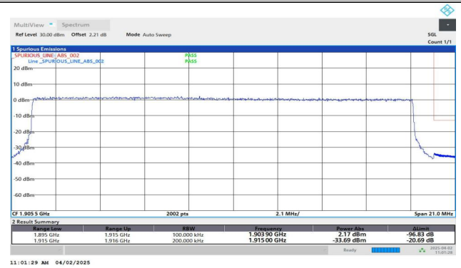
Band25-20MHz-QPSK-26590-100RB#0-PASS
