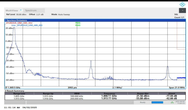
Band25-20MHz-QPSK-26590-1RB#0-PASS
