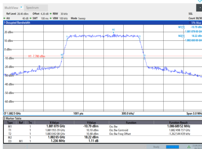
Band25-1.4MHz-QPSK-26365-6RB#0
