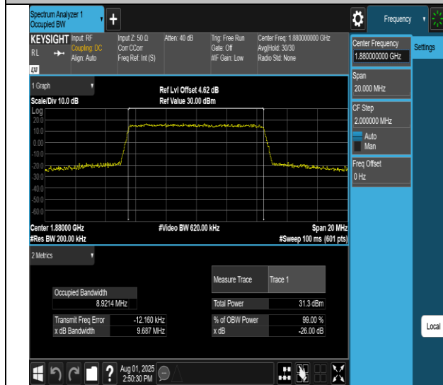
Band2-10MHz-16QAM-18800-50RB#0-PASS
