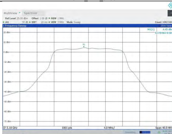
11a-CDD_Ant2_5180
