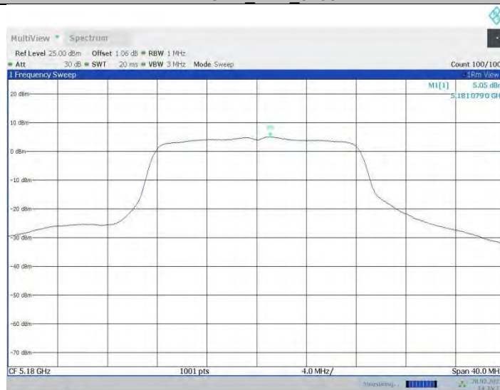
11a-CDD_Ant1_5180
