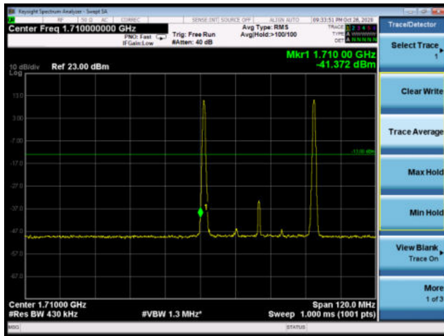
CA_66C QPSK 20MHz+20MHz CH-Low, 100%RB
