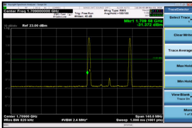
CA-4C-12A QPSK 20MHz+20MHz+20MHz CH-Low, 100%RB
