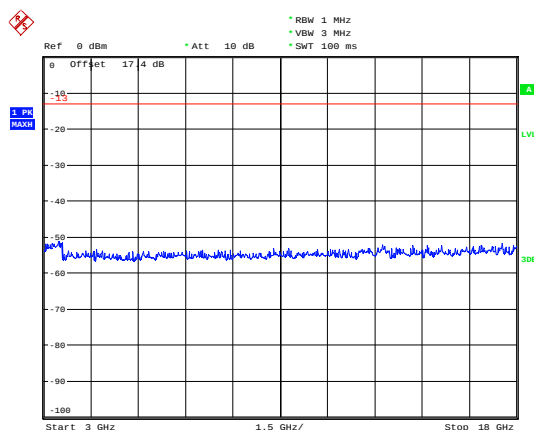
LTE Band 4 5MHz CH-Middle 3GHz~18GHz
