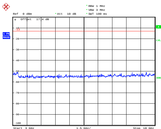
LTE Band 4 10MHz CH-Middle 3GHz~18GHz
