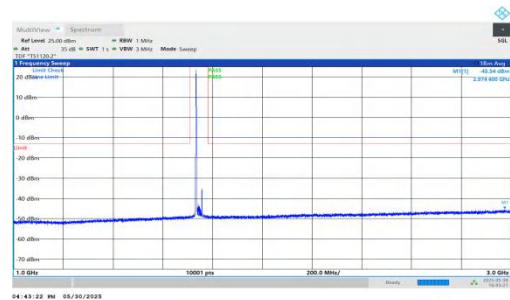
NTNV-n66-PC3-15-25-M-DFT-QPSK-Inner_1RB_Left-1000-3000-PASS
