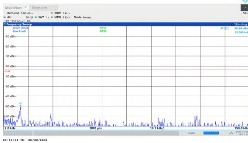
NTVN-n66-PC3-15-25-L-DFT-QPSK-Inner_1RB_Right-0.009-0.1-5-PASS
