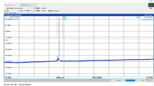
NTVN-n66-PC3-15-25-L-DFT-QPSK-Inner_1RB_Right-1000-3000-PASS
