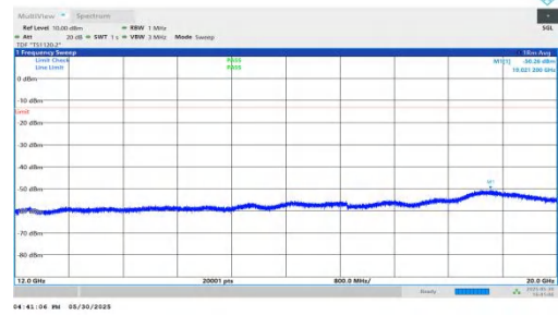
NTVN-n66-PC3-15-25-L-DFT-QPSK-Inner_1RB_Left-12000-20000-0-PASS
