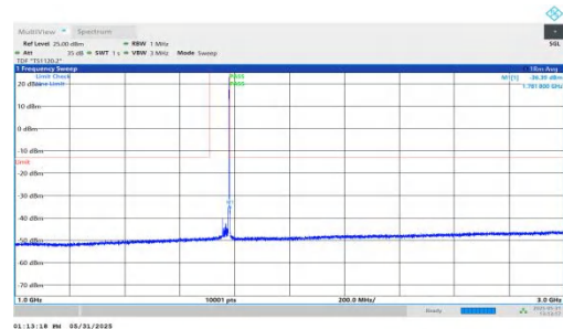
NTNV-n66-PC3-15-25-H-DFT-QPSK-Inner_1RB_Right-1000-3000 -PASS
