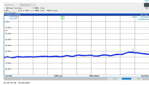
NTNV-n66-PC3-15-20-H-DFT-QPSK-Inner_1RB_Left-12000-2000 0-PASS
