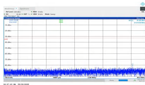
NTNV-n66-PC3-15-20-L-DFT-QPSK-Inner_1RB_Left-0.15-30-PAS S
