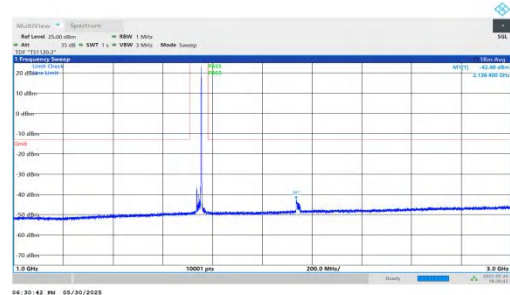
NTNV-n66-PC3-15-20-M-DFT-QPSK-Inner_1RB_Right-1000-3000 -PASS
