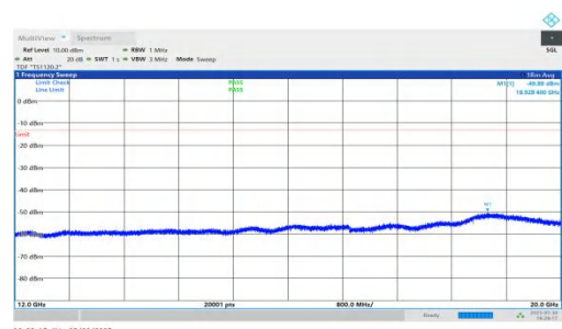
NTVN-n66-PC3-15-20-L-DFT-QPSK-Inner_1RB_Right-12000-20000 00-PASS
