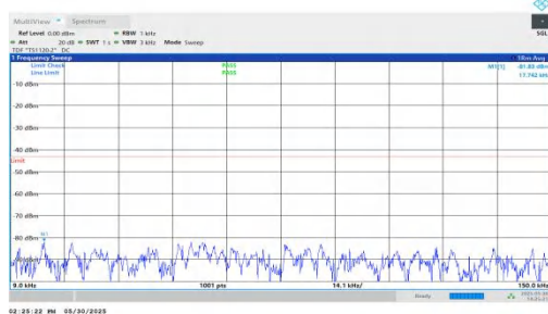
NTNV-n66-PC3-15-10-L-DFT-QPSK-Inner_1RB_Left-0.009-0.15-PASS
