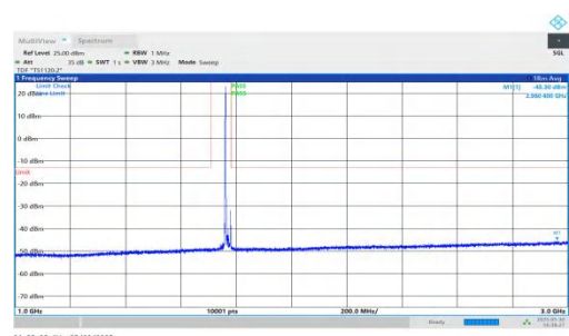
NTVN-n66-PC3-15-20-H-DFT-QPSK-Inner_1RB_Left-1000-3000-PASS
