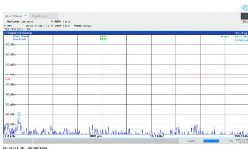
NTVN-n66-PC3-15-20-H-DFT-QPSK-Inner_1RB_Left-0.009-0.15-PASS
