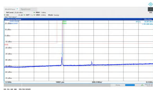
NTNV-n66-PC3-15-10-H-DFT-QPSK-Inner_1RB_Right-1000-3000- -PASS
