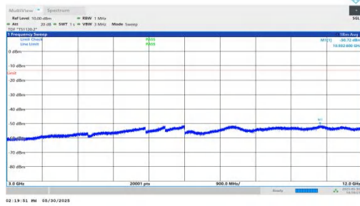
NTNV-n66-PC3-15-5-M-DFT-QPSK-Inner_1RB_Left-3000-12000 -PASS
