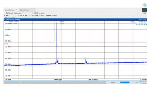
NTNV-n66-PC3-15-20-M-DFT-QPSK-Inner_1RB_Left-1000-3000-PASS
