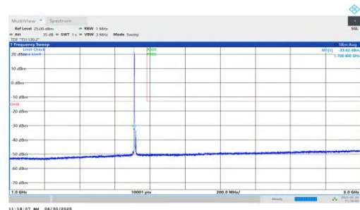
NTNV-n66-PC3-15-10-L-DFT-QPSK-Inner_1RB_Left-1000-3000-PASS
