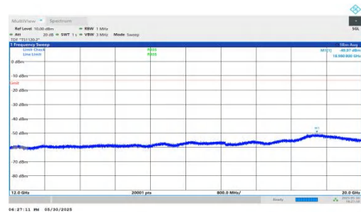
NTNV-n66-PC3-15-20-L-DFT-BPSK-Inner_1RB_Right-12000-200 00-PASS
