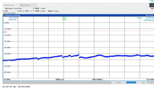
NTNV-n66-PC3-15-10-M-DFT-QPSK-Inner_1RB_Left-3000-1200 0-PASS
