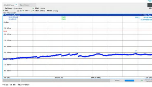
NTNV-n66-PC3-15-15-M-DFT-QPSK-Inner_1RB_Left-3000-1200 0-PASS
