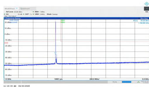
NTNV-n66-PC3-15-15-L-DFT-QPSK-Inner_1RB_Left-1000-3000-P ASS
