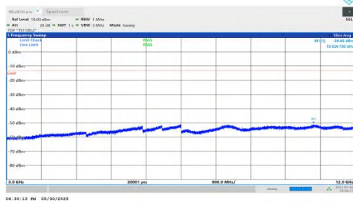
NTNV-n66-PC3-15-20-M-DFT-QPSK-Inner_1RB_Left-3000-1200 0-PASS
