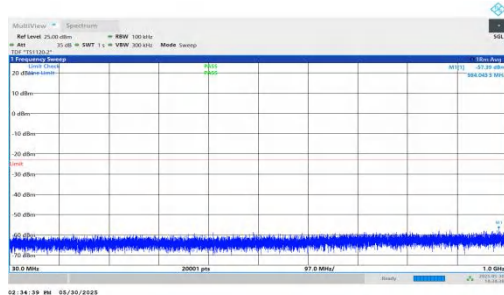
NTVN-n66-PC3-15-15-L-DFT-QPSK-Inner_1RB_Right-30-1000-P ASS
