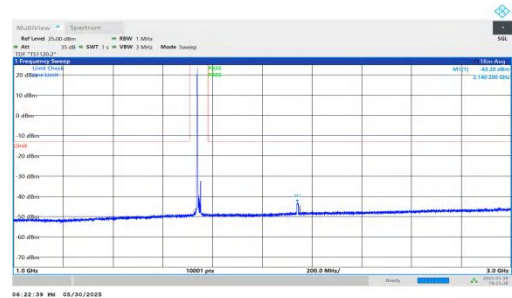
NTNV-n66-PC3-15-15-M-DFT-QPSK-Inner_1RB_Left-1000-3000-PASS
