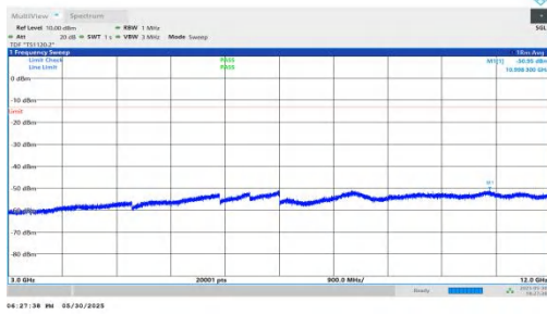
NTVN-n66-PC3-15-20-L-DFT-QPSK-Inner_1RB_Left-3000-12000 -PASS
