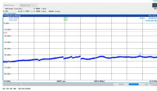
NTVN-n66-PC3-15-15-L-DFT-QPSK-Inner_1RB_Left-3000-12000 -PASS
