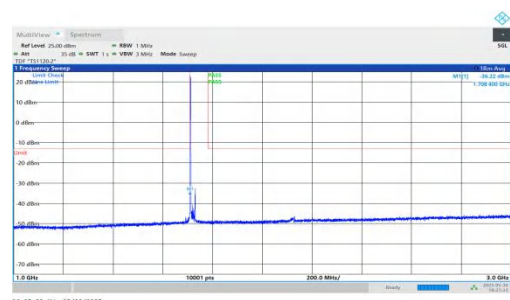
NTNV-n66-PC3-15-20-L-DFT-QPSK-Inner_1RB_Left-1000-3000-P ASS
