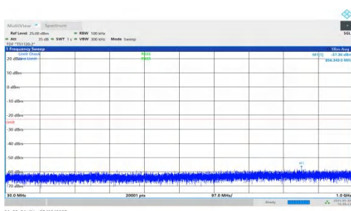
NTVN-n66-PC3-15-20-H-DFT-QPSK-Inner_1RB_Left-30-1000-PASS
