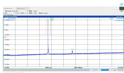
NTNV-n66-PC3-15-10-M-DFT-QPSK-Inner_1RB_Left-1000-3000-PASS
