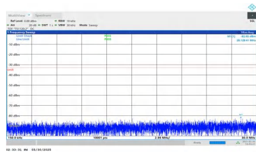
NTNV-n66-PC3-15-15-L-DFT-QPSK-Inner_1RB_Left-0.15-30-PAS S
