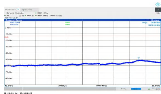
NTNV-n66-PC3-15-10-L-DFT-BPSK-Inner_1RB_Left-12000-20000 -PASS
