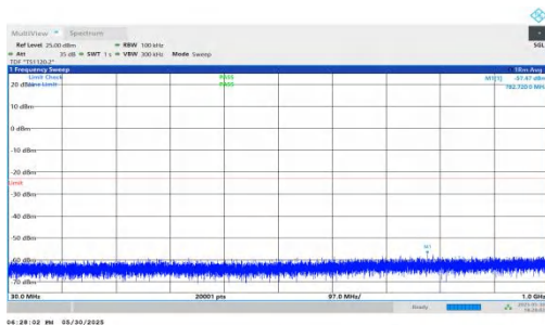
NTVN-n66-PC3-15-20-L-DFT-QPSK-Inner_1RB_Right-30-1000-P ASS
