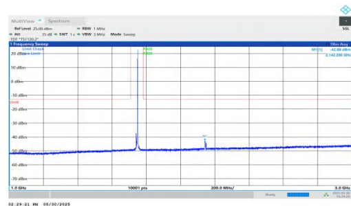
NTNV-n66-PC3-15-10-M-DFT-QPSK-Inner_1RB_Right-1000-3000- -PASS
