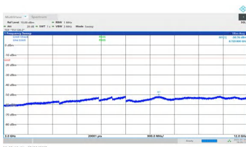
NTVN-n66-PC3-15-20-L-DFT-QPSK-Inner_1RB_Right-3000-12000 00-PASS
