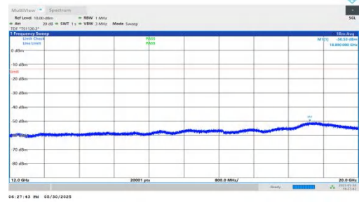
NTVN-n66-PC3-15-20-L-DFT-QPSK-Inner_1RB_Left-12000-2000 0-PASS
