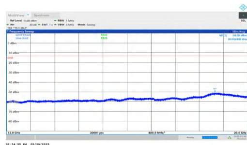
NTVN-n66-PC3-15-15-L-DFT-QPSK-Inner_1RB_Right-12000-20000 00-PASS
