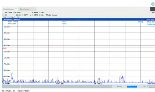
NTVN-n66-PC3-15-20-L-DFT-QPSK-Inner_1RB_Right-0.009-0.1 5-PASS
