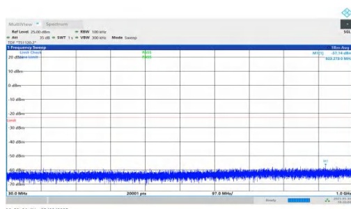
NTNV-n66-PC3-15-20-M-DFT-QPSK-Inner_1RB_Left-30-1000-PASS
