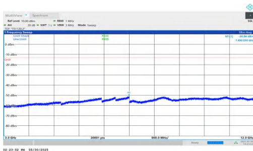
NTNV-n66-PC3-15-10-L-DFT-BPSK-Inner_1RB_Left-3000-12000 -PASS
