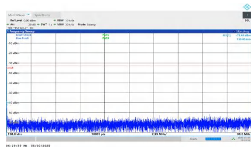
NTNV-n66-PC3-15-20-M-DFT-QPSK-Inner_1RB_Left-0.15-30-PASS
