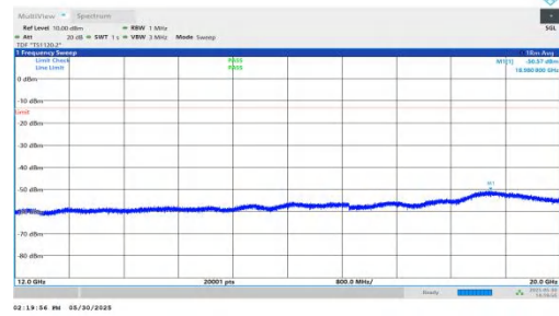
NTNV-n66-PC3-15-5-M-DFT-QPSK-Inner_1RB_Left-12000-20000 -PASS
