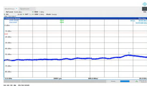
NTNV-n66-PC3-15-20-L-DFT-BPSK-Inner_1RB_Left-12000-20000-PASS
