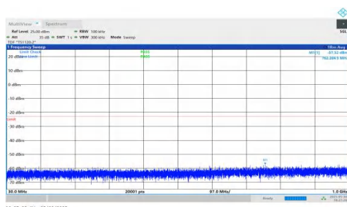
NTNV-n66-PC3-15-20-L-DFT-QPSK-Inner_1RB_Left-30-1000-P ASS
