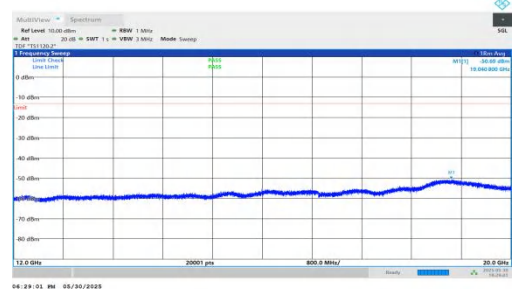
NTNV-n66-PC3-15-20-M-DFT-BPSK-Inner_1RB_Left-12000-20000-PASS
