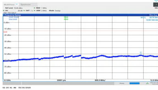
NTNV-n66-PC3-15-10-L-DFT-QPSK-Inner_1RB_Left-3000-12000 -PASS
