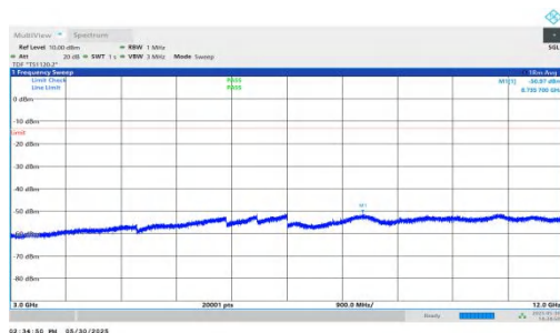
NTVN-n66-PC3-15-15-L-DFT-QPSK-Inner_1RB_Right-3000-12000 00-PASS
