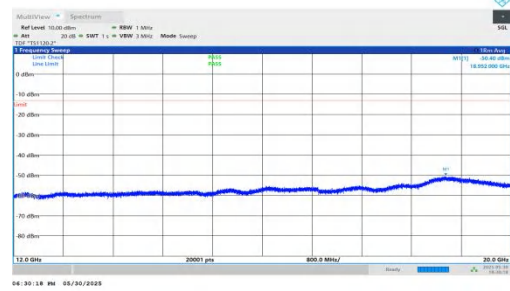
NTNV-n66-PC3-15-20-M-DFT-QPSK-Inner_1RB_Left-12000-2000 0-PASS
