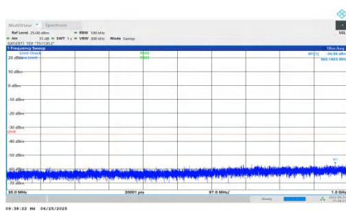
NTVN-n41-PC2-30-60-H-DFT-QPSK-Inner_1RB_Left-30-1000-P ASS
