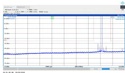
NTNV-n41-PC2-30-70-M-DFT-QPSK-Inner_1RB_Right-1000-3000- -PASS
