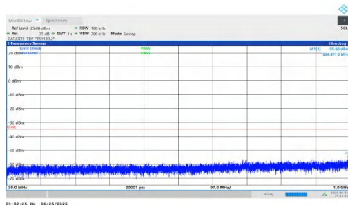
NTNV-n41-PC2-30-60-M-DFT-QPSK-Inner_1RB_Left-30-1000-PASS
