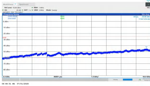
NTVN-n41-PC2-30-60-L-DFT-QPSK-Inner_1RB_Left-3000-18000 -PASS
