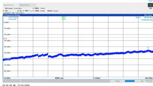
NTVN-n41-PC2-30-80-L-DFT-QPSK-Inner_1RB_Left-3000-18000 -PASS
