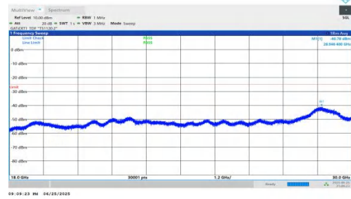
NTVN-n41-PC2-30-50-L-DFT-QPSK-Inner_1RB_Left-18000-3000 0-PASS
