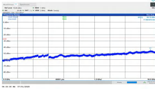
NTVN-n41-PC2-30-45-L-DFT-QPSK-Inner_1RB_Left-3000-18000 -PASS
