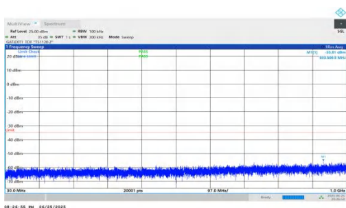
NTVN-n41-PC2-30-35-H-DFT-QPSK-Inner_1RB_Left-30-1000-P ASS
