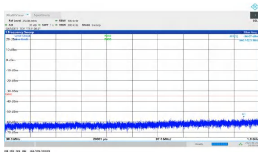
NTNV-n41-PC2-30-35-M-DFT-QPSK-Inner_1RB_Left-30-1000-PASS
