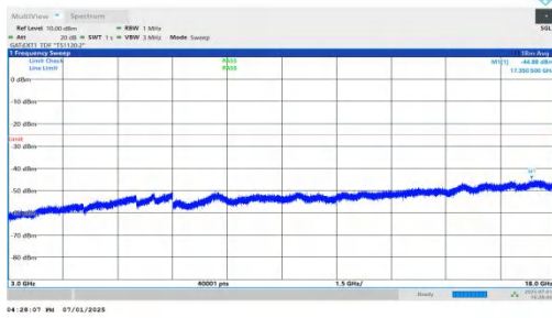
NTVN-n41-PC2-30-40-L-DFT-QPSK-Inner_1RB_Left-3000-18000 -PASS
