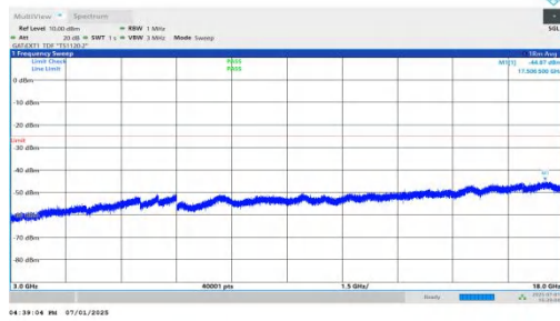
NTVN-n41-PC2-30-50-L-DFT-QPSK-Inner_1RB_Left-3000-18000 -PASS
