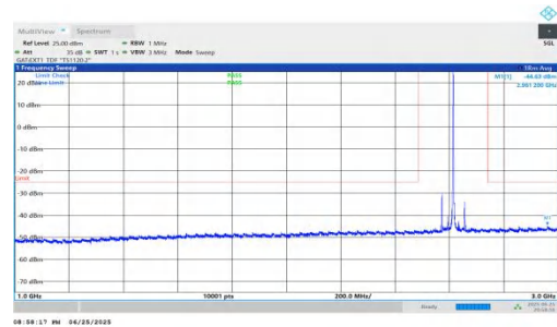
NTNV-n41-PC2-30-45-M-DFT-QPSK-Inner_1RB_Right-1000-3000- -PASS
