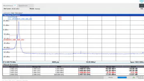
NTNV-n41-PC2-30-90-L-DFT-BPSK-Edge 1RB Left
