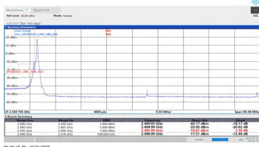
NTNV-n41-PC2-30-80-L-DFT-BPSK-Edge 1RB Left
