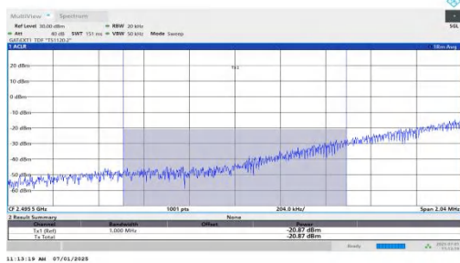
NTNV-n41-PC2-30-100-L-DFT-QPSK-Edge_1RB_Left-PASS
