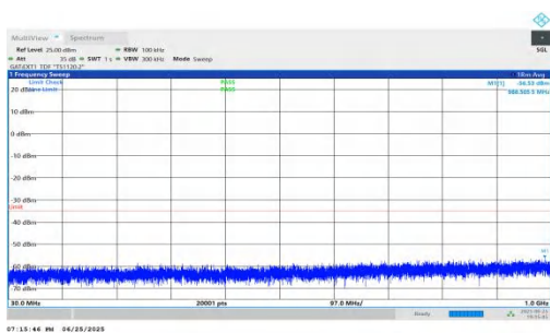
NTVN-n41-PC2-30-15-H-DFT-QPSK-Inner_1RB_Left-30-1000-P ASS
