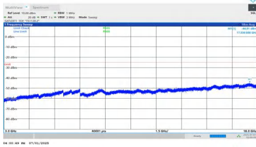
NTVN-n41-PC2-30-15-L-DFT-QPSK-Inner_1RB_Left-3000-18000 -PASS
