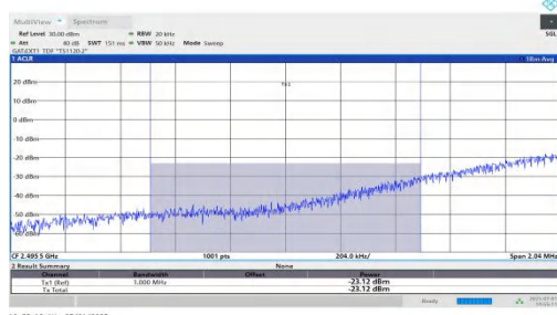
NTNV-n41-PC2-30-90-L-DFT-BPSK-Edge 1RB Left-PASS
