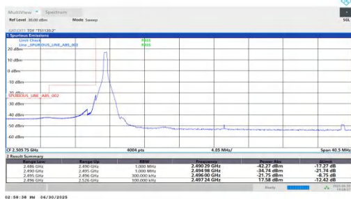
NTNV-n41-PC2-30-30-L-DFT-QPSK-Edge_1RB_Left-PASS
