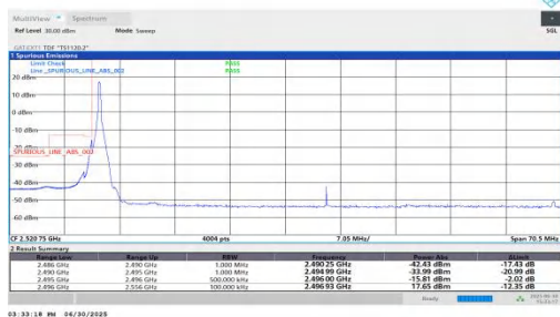
NTNV-n41-PC2-30-60-L-DFT-BPSK-Edge 1RB Left-PASS
