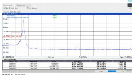
NTNV-n41-PC2-30-60-L-DFT-QPSK-Edge 1RB Left-PASS
