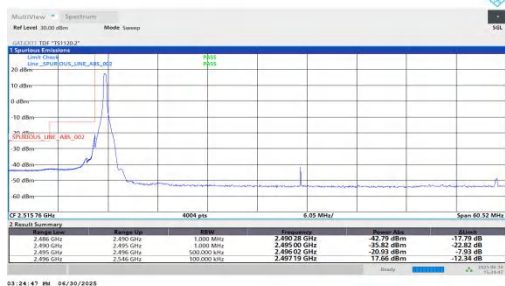
NTNV-n41-PC2-30-50-L-DFT-BPSK-Edge 1RB Left-PASS
