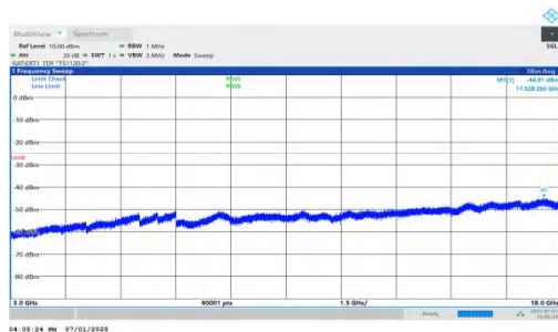
NTNV-n41-PC2-30-20-L-DFT-BPSK-Inner_1RB_Left-3000-18000 -PASS
