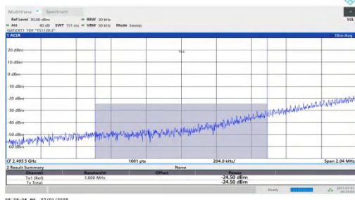
NTNV-n41-PC2-30-80-L-DFT-QPSK-Edge_1RB_Left-PASS
