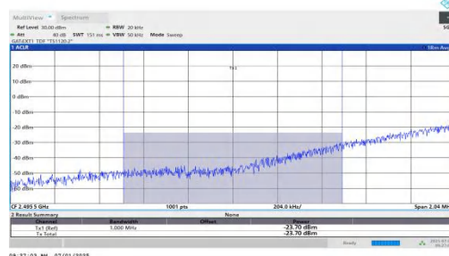
NTNV-n41-PC2-30-80-L-DFT-BPSK-Edge 1RB Left-PASS
