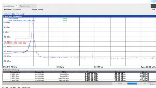
NTNV-n41-PC2-30-50-L-DFT-QPSK-Edge 1RB Left-PASS
