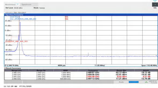
NTNV-n41-PC2-30-100-L-DFT-QPSK-Edge_1RB_Left
