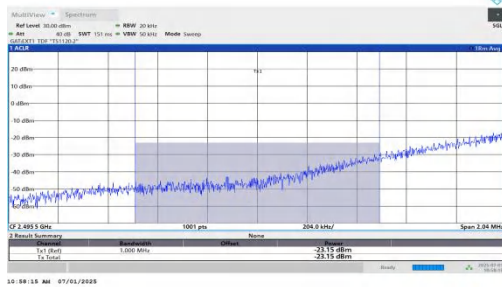
NTNV-n41-PC2-30-90-L-DFT-QPSK-Edge_1RB_Left-PASS
