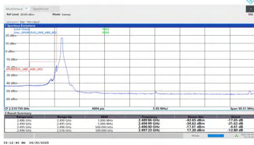
NTNV-n41-PC2-30-40-L-DFT-QPSK-Edge_1RB_Left-PASS
