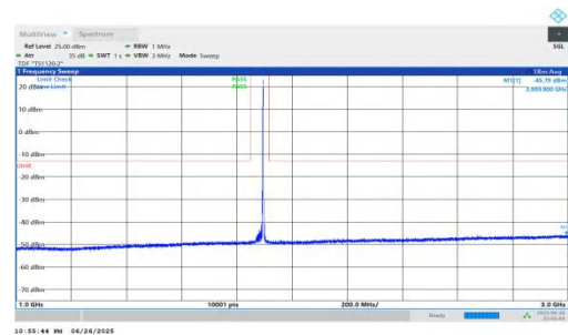
NTNV-n25-PC3-15-25-M-DFT-QPSK-Inner_1RB_Right-1000-3000- -PASS
