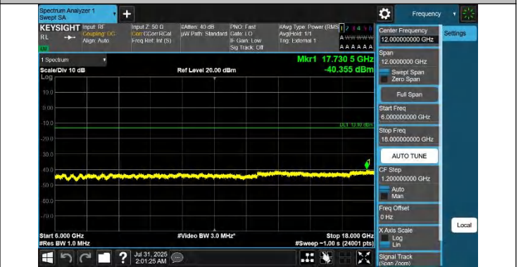
42-42-20MHz-10MHz-QPSK-QPSK-42891-43035-1RB#0-0RB#0- 6000~18000MHz-PASS
