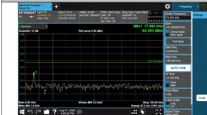
42-42-20MHz-10MHz-QPSK-QPSK-42891-43035-1RB#99-0RB# 0-0.009~0.15MHz-PASS
