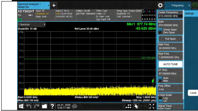
42-42-20MHz-10MHz-QPSK-QPSK-42891-43035-1RB#99-0RB# 0-30~1000MHz-PASS
