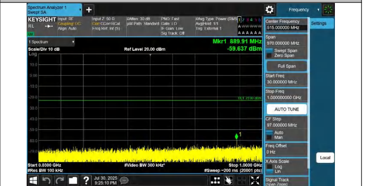
42-42-10MHz-20MHz-QPSK-QPSK-42145-42289-1RB#0-0RB#0-30~1000MHz-PASS
