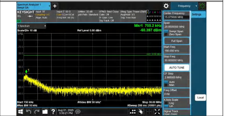
42-42-5MHz-20MHz-QPSK-QPSK-42873-42990-1RB#24-0RB#0- 0.15~30MHz-PASS
