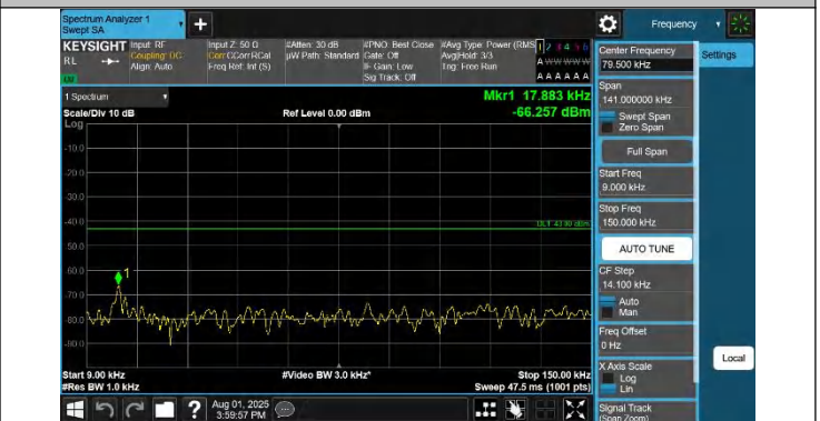
42-42-10MHz-20MHz-QPSK-QPSK-42145-42289-1RB#49-0RB# 0-0.009~0.15MHz-PASS
