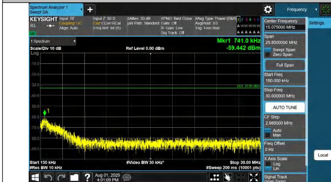
42-42-10MHz-20MHz-QPSK-QPSK-42846-42990-1RB#0-0RB#0- 0.15~30MHz-PASS
