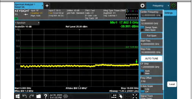
42-42-5MHz-20MHz-QPSK-QPSK-42873-42990-1RB#24-0RB#0- 6000~18000MHz-PASS
