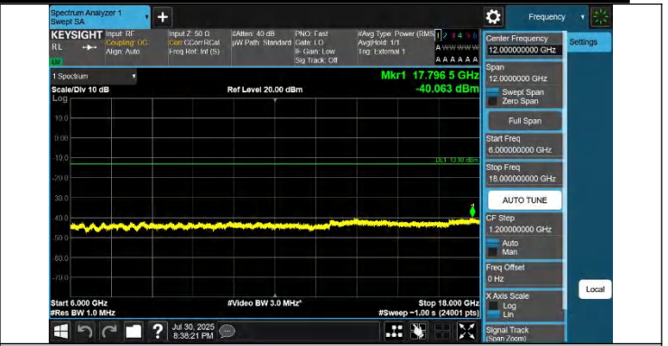
42-42-5MHz-20MHz-QPSK-QPSK-42873-42990-1RB#0-0RB#0-6 000~18000MHz-PASS
