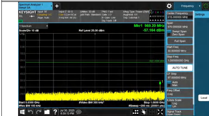
42-42-5MHz-20MHz-QPSK-QPSK-42873-42990-1RB#24-0RB#0- 30~1000MHz-PASS
