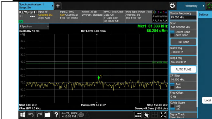
66-66-20MHz-5MHz-QPSK-QPSK-132072-132189-1RB#0-0RB# 0-0.009~0.15MHz-PASS
