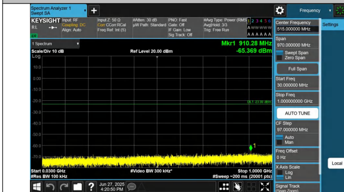
66-66-20MHz-5MHz-QPSK-QPSK-132397-132514-1RB#0-1RB# 24-30~1000MHz-PASS
