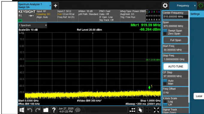
66-66-15MHz-20MHz-QPSK-QPSK-132401-132572-1RB#0-1RB #99-30~1000MHz-PASS
