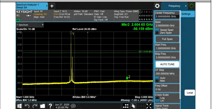
66-66-20MHz-5MHz-QPSK-QPSK-132397-132514-1RB#0-1RB# 24-1000~3000MHz-PASS
