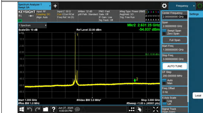
66-66-15MHz-20MHz-QPSK-QPSK-132401-132572-1RB#0-0RB #0-1000~3000MHz-PASS
