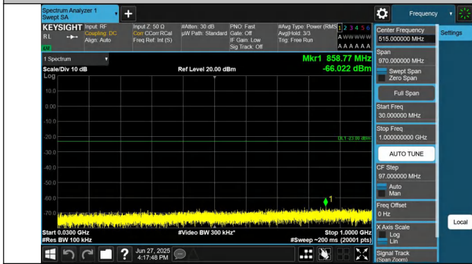
66-66-20MHz-5MHz-QPSK-QPSK-132072-132189-1RB#99-0RB #0-30~1000MHz-PASS
