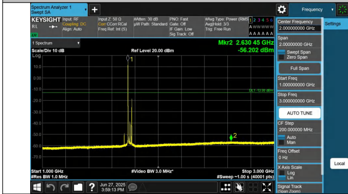
66-66-15MHz-20MHz-QPSK-QPSK-132325-132496-1RB#0-1RB #99-1000~3000MHz-PASS
