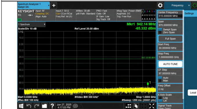
66-66-20MHz-5MHz-QPSK-QPSK-132072-132189-1RB#0-0RB# 0-30~1000MHz-PASS
