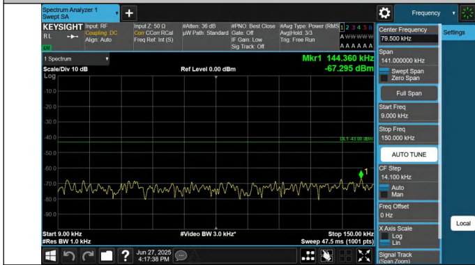
66-66-20MHz-5MHz-QPSK-QPSK-132072-132189-1RB#99-0RB #0-0.009~0.15MHz-PASS
