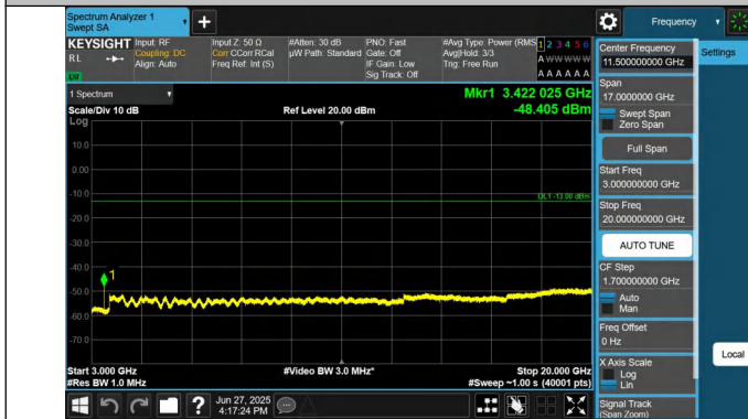
66-66-20MHz-5MHz-QPSK-QPSK-132072-132189-1RB#0-0RB# 0-3000~20000MHz-PASS
