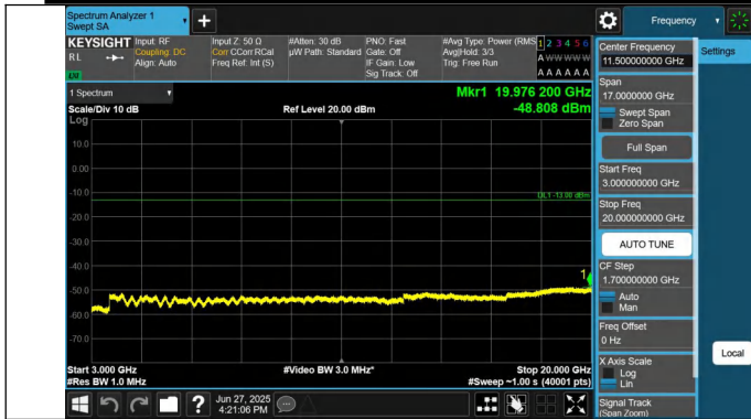
66-66-20MHz-5MHz-QPSK-QPSK-132397-132514-1RB#0-1RB# 24-3000~20000MHz-PASS
