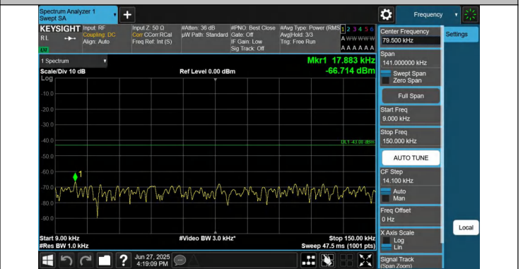
66-66-20MHz-5MHz-QPSK-QPSK-132397-132514-1RB#0-0RB# 0-0.009~0.15MHz-PASS
