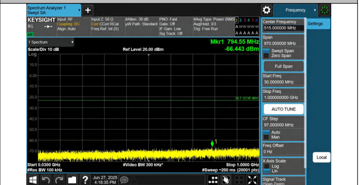
66-66-20MHz-5MHz-QPSK-QPSK-132072-132189-1RB#0-1RB# 24-30~1000MHz-PASS
