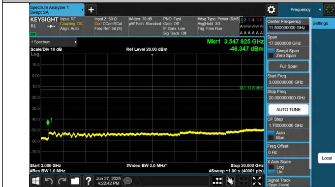
66-66-20MHz-5MHz-QPSK-QPSK-132522-132639-1RB#99-0RB #0-3000~20000MHz-PASS
