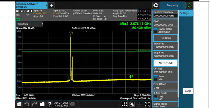
66-66-15MHz-20MHz-QPSK-QPSK-132401-132572-1RB#0-1RB #99-1000~3000MHz-PASS
