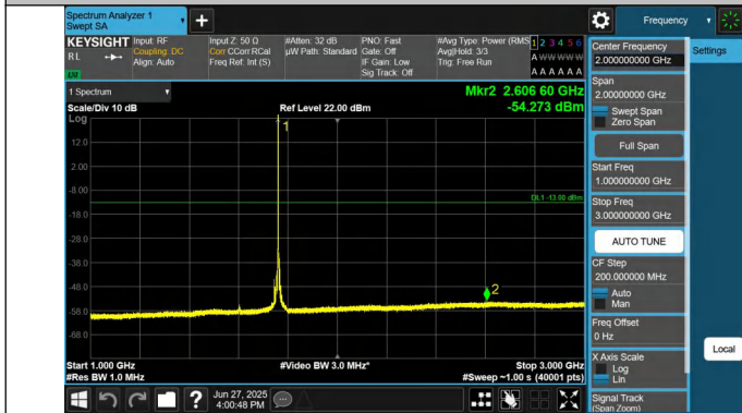
66-66-15MHz-20MHz-QPSK-QPSK-132401-132572-1RB#74-0R B#0-1000~3000MHz-PASS
