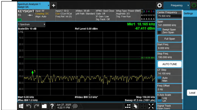
66-66-20MHz-5MHz-QPSK-QPSK-132522-132639-1RB#99-0RB #0-0.009~0.15MHz-PASS
