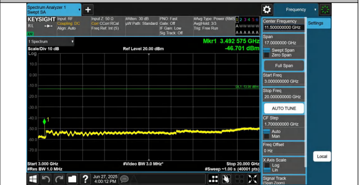
66-66-15MHz-20MHz-QPSK-QPSK-132401-132572-1RB#0-0RB #0-3000~20000MHz-PASS
