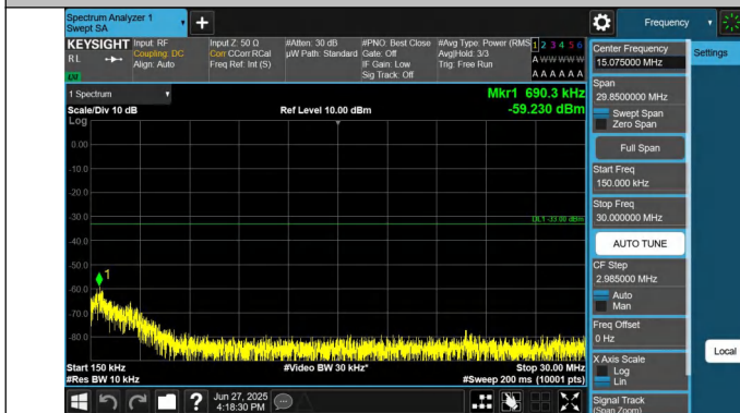
66-66-20MHz-5MHz-QPSK-QPSK-132072-132189-1RB#0-1RB# 24-0.15~30MHz-PASS
