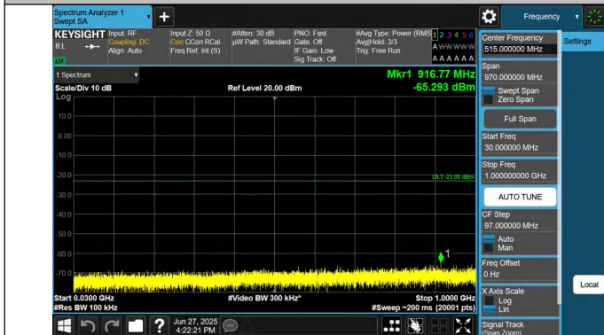
66-66-20MHz-5MHz-QPSK-QPSK-132522-132639-1RB#99-0RB #0-30~1000MHz-PASS
