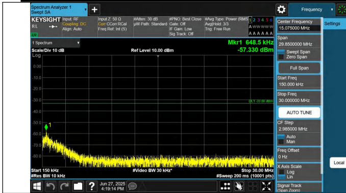
66-66-20MHz-5MHz-QPSK-QPSK-132397-132514-1RB#0-0RB# 0-0.15~30MHz-PASS
