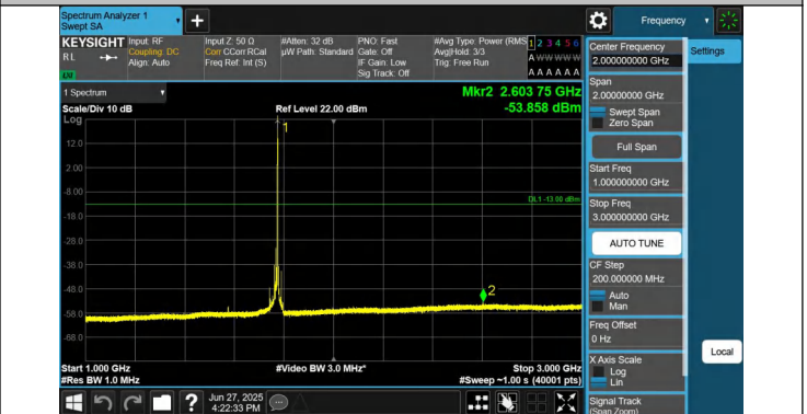
66-66-20MHz-5MHz-QPSK-QPSK-132522-132639-1RB#99-0RB #0-1000~3000MHz-PASS
