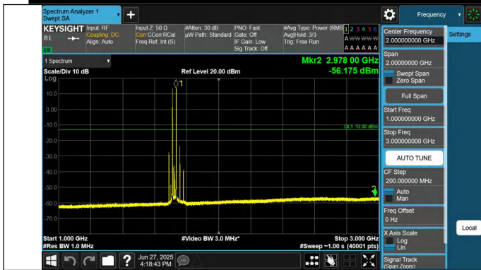
66-66-20MHz-5MHz-QPSK-QPSK-132072-132189-1RB#0-1RB# 24-1000~3000MHz-PASS
