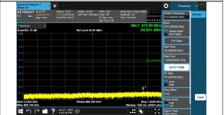
66-66-15MHz-20MHz-QPSK-QPSK-132401-132572-1RB#74-0R B#0-30~1000MHz-PASS
