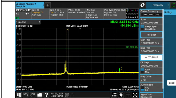
66-66-20MHz-5MHz-QPSK-QPSK-132397-132514-1RB#99-0RB #0-1000~3000MHz-PASS
