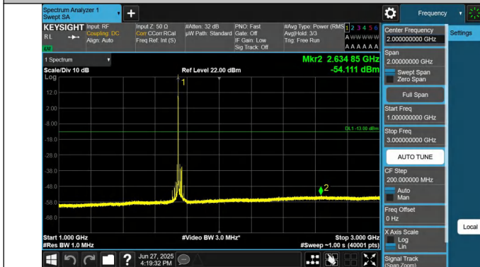
66-66-20MHz-5MHz-QPSK-QPSK-132397-132514-1RB#0-0RB# 0-1000~3000MHz-PASS
