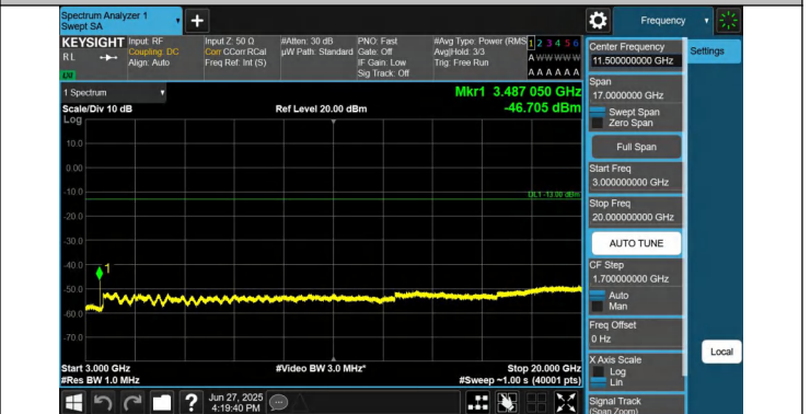
66-66-20MHz-5MHz-QPSK-QPSK-132397-132514-1RB#0-0RB# 0-3000~20000MHz-PASS
