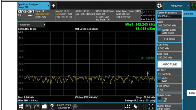
66-66-20MHz-5MHz-QPSK-QPSK-132397-132514-1RB#0-1RB# 24-0.009~0.15MHz-PASS
