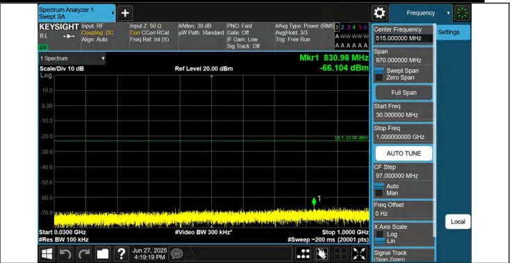
66-66-20MHz-5MHz-QPSK-QPSK-132397-132514-1RB#0-0RB# 0-30~1000MHz-PASS
