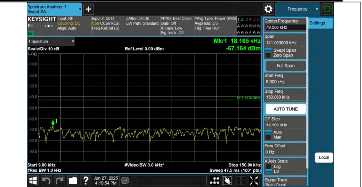
66-66-20MHz-5MHz-QPSK-QPSK-132397-132514-1RB#99-0RB #0-0.009~0.15MHz-PASS
