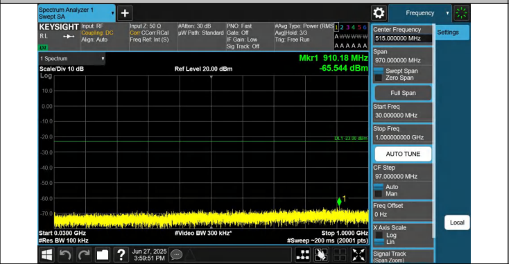
66-66-15MHz-20MHz-QPSK-QPSK-132401-132572-1RB#0-0RB #0-30~1000MHz-PASS
