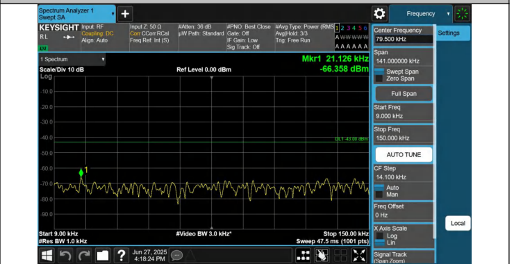
66-66-20MHz-5MHz-QPSK-QPSK-132072-132189-1RB#0-1RB# 24-0.009~0.15MHz-PASS
