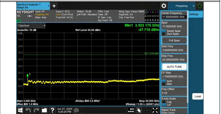
66-66-20MHz-5MHz-QPSK-QPSK-132397-132514-1RB#99-0RB #0-3000~20000MHz-PASS
