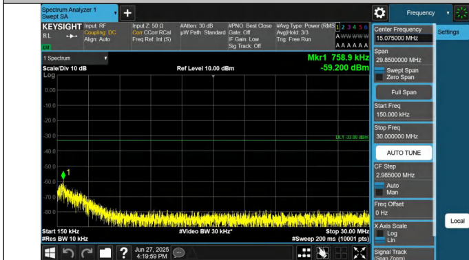
66-66-20MHz-5MHz-QPSK-QPSK-132397-132514-1RB#99-0RB #0-0.15~30MHz-PASS
