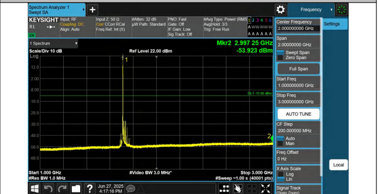
66-66-20MHz-5MHz-QPSK-QPSK-132072-132189-1RB#0-0RB# 0-1000~3000MHz-PASS
