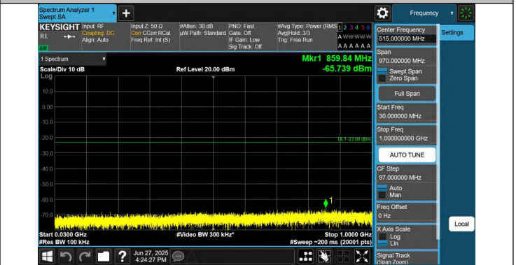
66-66-20MHz-10MHz-QPSK-QPSK-132072-132216-1RB#0-0RB #0-30~1000MHz-PASS
