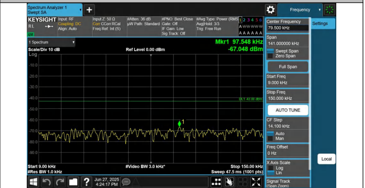
66-66-20MHz-10MHz-QPSK-QPSK-132072-132216-1RB#0-0RB #0-0.009~0.15MHz-PASS
