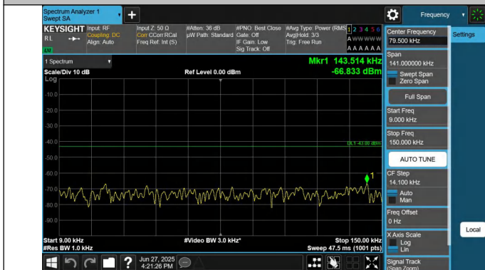
66-66-20MHz-5MHz-QPSK-QPSK-132522-132639-1RB#0-0RB# 0-0.009~0.15MHz-PASS
