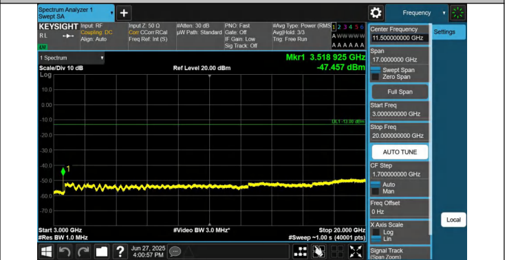
66-66-15MHz-20MHz-QPSK-QPSK-132401-132572-1RB#74-0R B#0-3000~20000MHz-PASS
