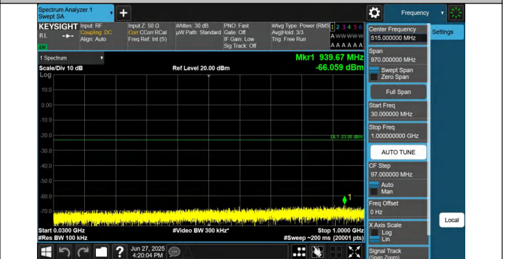
66-66-20MHz-5MHz-QPSK-QPSK-132397-132514-1RB#99-0RB #0-30~1000MHz-PASS
