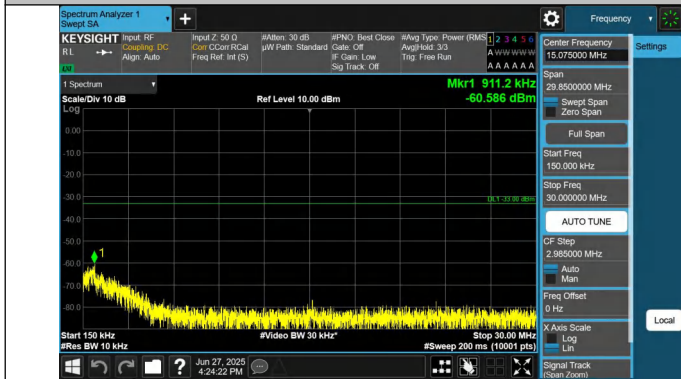
66-66-20MHz-10MHz-QPSK-QPSK-132072-132216-1RB#0-0RB #0-0.15~30MHz-PASS
