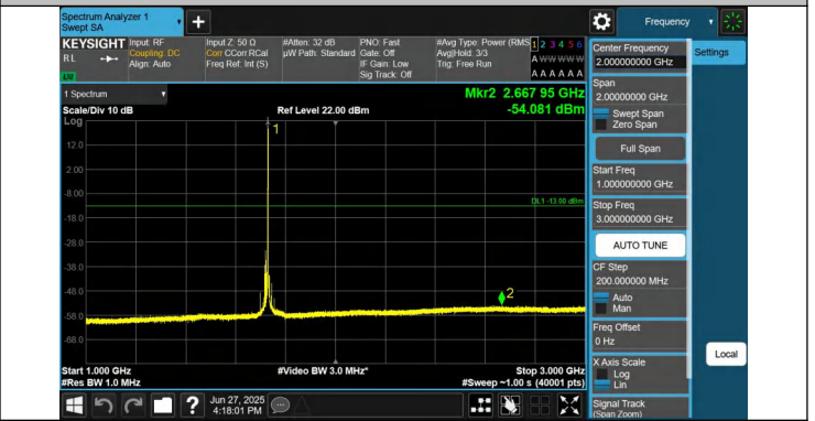
66-66-20MHz-5MHz-QPSK-QPSK-132072-132189-1RB#99-0RB #0-1000~3000MHz-PASS
