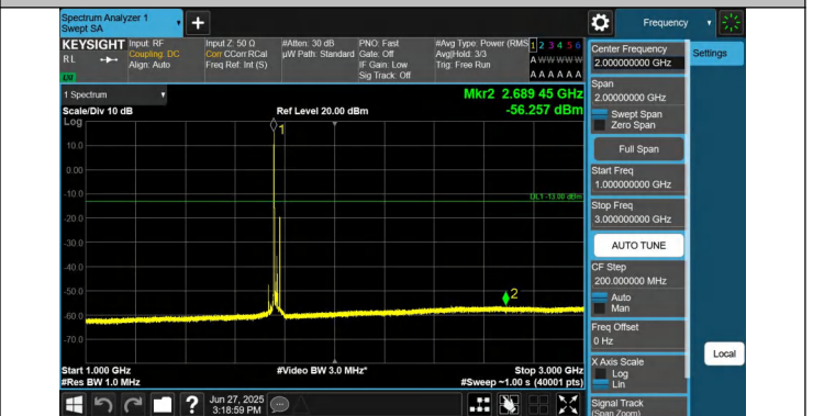
66-66-15MHz-10MHz-QPSK-QPSK-132499-132619-1RB#0-1RB #49-1000~3000MHz-PASS
