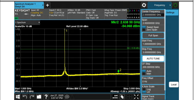
66-66-15MHz-20MHz-QPSK-QPSK-132325-132496-1RB#0-0RB #0-1000~3000MHz-PASS
