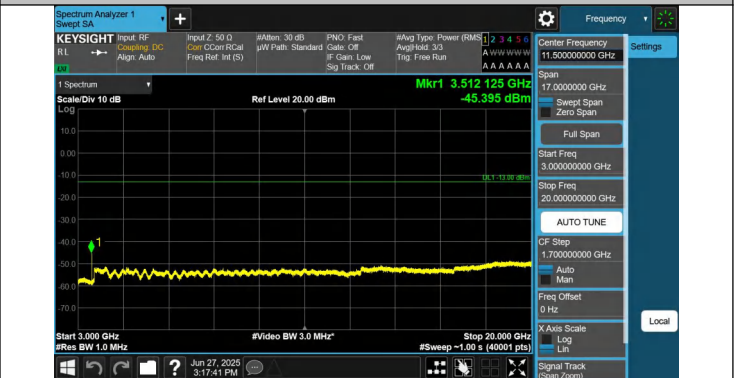
66-66-15MHz-10MHz-QPSK-QPSK-132499-132619-1RB#0-0RB #0-3000~20000MHz-PASS
