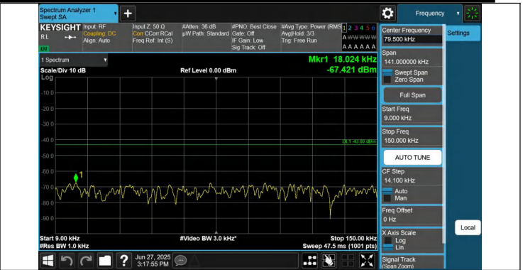
66-66-15MHz-10MHz-QPSK-QPSK-132499-132619-1RB#74-0R B#0-0.009~0.15MHz-PASS
