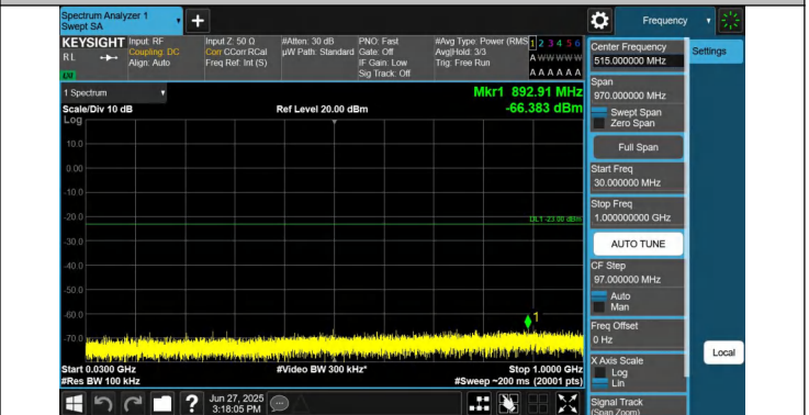
66-66-15MHz-10MHz-QPSK-QPSK-132499-132619-1RB#74-0R B#0-30~1000MHz-PASS
