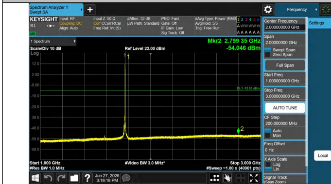
66-66-15MHz-10MHz-QPSK-QPSK-132499-132619-1RB#74-0R B#0-1000~3000MHz-PASS
