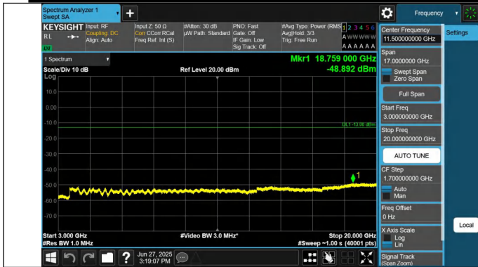
66-66-15MHz-10MHz-QPSK-QPSK-132499-132619-1RB#0-1RB #49-3000~20000MHz-PASS
