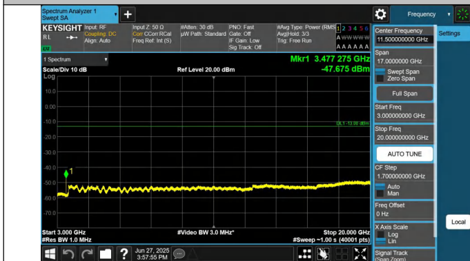
66-66-15MHz-20MHz-QPSK-QPSK-132325-132496-1RB#0-0RB #0-3000~20000MHz-PASS
