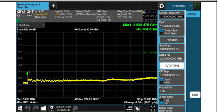
66-66-15MHz-10MHz-QPSK-QPSK-132499-132619-1RB#74-0R B#0-3000~20000MHz-PASS
