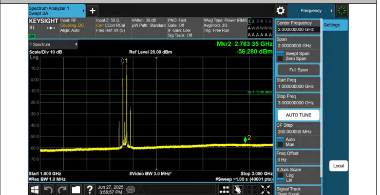
66-66-15MHz-20MHz-QPSK-QPSK-132050-132221-1RB#0-1RB #99-1000~3000MHz-PASS
