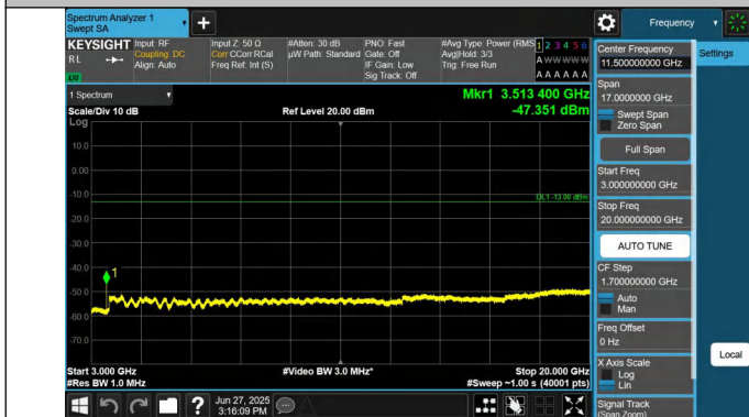
66-66-15MHz-10MHz-QPSK-QPSK-132373-132493-1RB#74-0R B#0-3000~20000MHz-PASS
