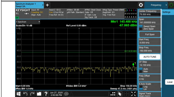
66-66-10MHz-20MHz-QPSK-QPSK-132027-132171-1RB#0-0RB #0-0.009~0.15MHz-PASS
