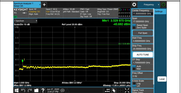
66-66-10MHz-15MHz-QPSK-QPSK-132477-132597-1RB#49-0R B#0-3000~20000MHz-PASS
