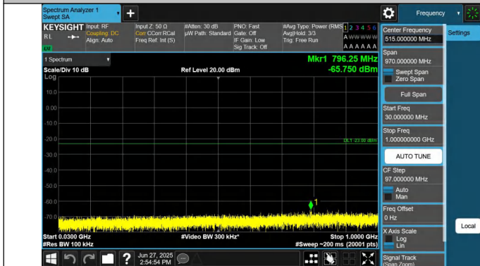
66-66-10MHz-20MHz-QPSK-QPSK-132328-132472-1RB#0-1RB #99-30~1000MHz-PASS
