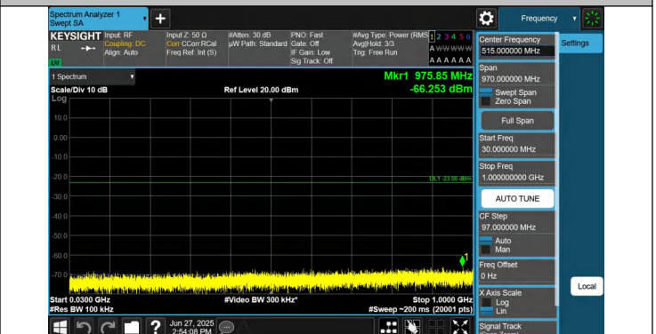
66-66-10MHz-20MHz-QPSK-QPSK-132328-132472-1RB#49-0R B#0-30~1000MHz-PASS
