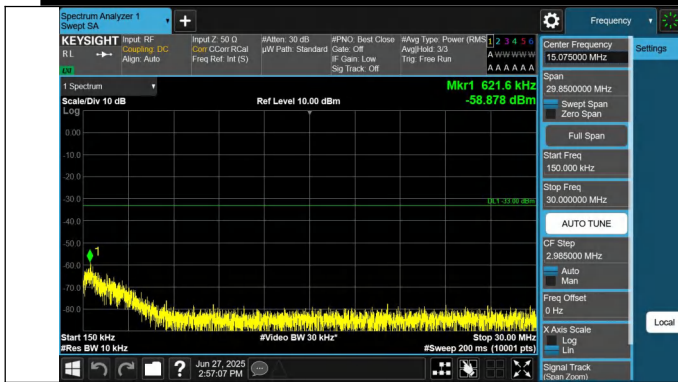
66-66-10MHz-20MHz-QPSK-QPSK-132428-132572-1RB#0-1RB #99-0.15~30MHz-PASS
