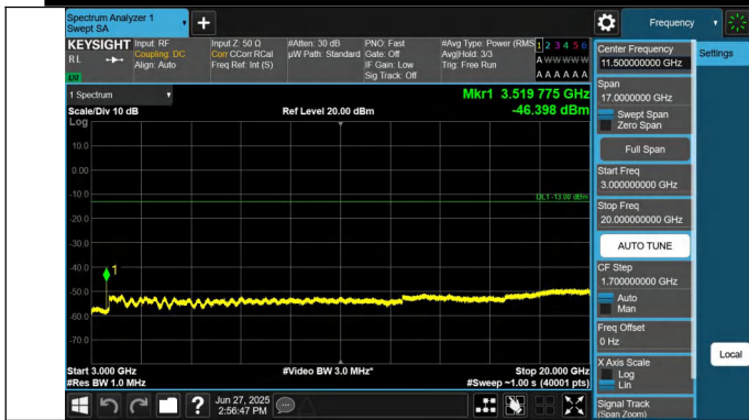
66-66-10MHz-20MHz-QPSK-QPSK-132428-132572-1RB#49-0R B#0-3000~20000MHz-PASS
