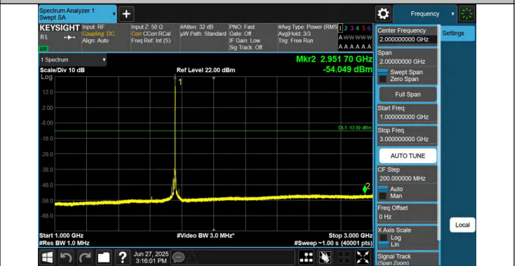
66-66-15MHz-10MHz-QPSK-QPSK-132373-132493-1RB#74-0R B#0-1000~3000MHz-PASS
