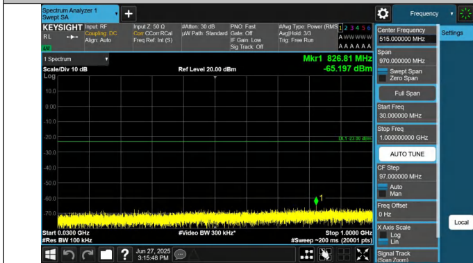
66-66-15MHz-10MHz-QPSK-QPSK-132373-132493-1RB#74-0R B#0-30~1000MHz-PASS
