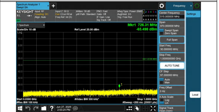
66-66-10MHz-20MHz-QPSK-QPSK-132328-132472-1RB#0-0RB #0-30~1000MHz-PASS
