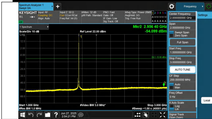
66-66-10MHz-20MHz-QPSK-QPSK-132328-132472-1RB#49-0R B#0-1000~3000MHz-PASS
