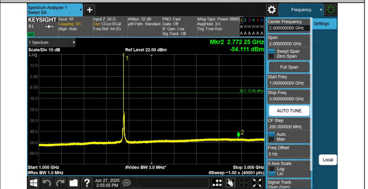
66-66-10MHz-20MHz-QPSK-QPSK-132428-132572-1RB#0-0RB #0-1000~3000MHz-PASS
