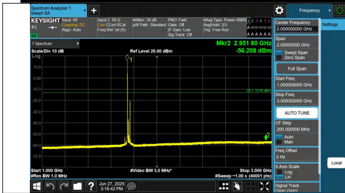
66-66-15MHz-10MHz-QPSK-QPSK-132373-132493-1RB#0-1RB #49-1000~3000MHz-PASS
