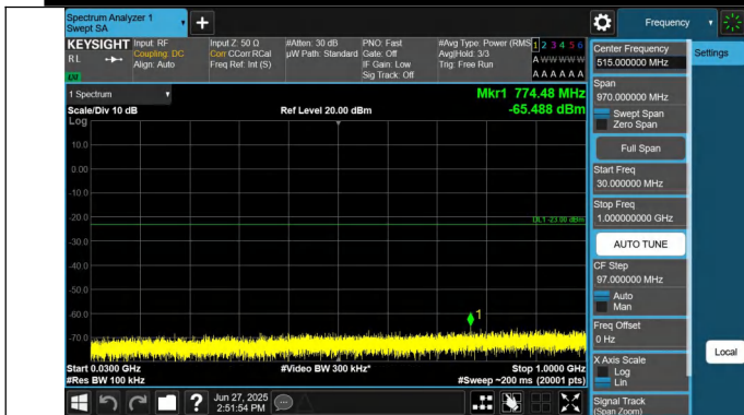
66-66-10MHz-20MHz-QPSK-QPSK-132027-132171-1RB#49-0R B#0-30~1000MHz-PASS
