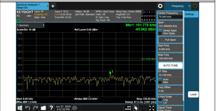
66-66-10MHz-20MHz-QPSK-QPSK-132428-132572-1RB#0-1RB #99-0.009~0.15MHz-PASS
