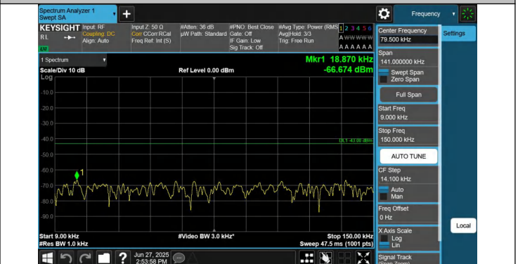
66-66-10MHz-20MHz-QPSK-QPSK-132328-132472-1RB#49-0R B#0-0.009~0.15MHz-PASS
