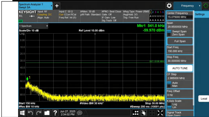
66-66-10MHz-15MHz-QPSK-QPSK-132477-132597-1RB#49-0R B#0-0.15~30MHz-PASS
