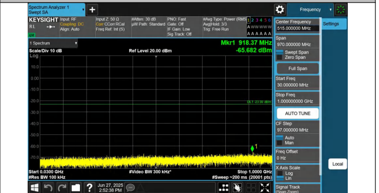
66-66-10MHz-20MHz-QPSK-QPSK-132027-132171-1RB#0-1RB #99-30~1000MHz-PASS
