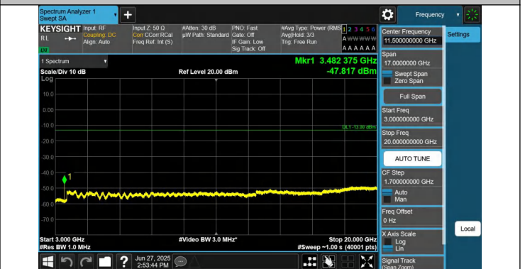
66-66-10MHz-20MHz-QPSK-QPSK-132328-132472-1RB#0-0RB #0-3000~20000MHz-PASS
