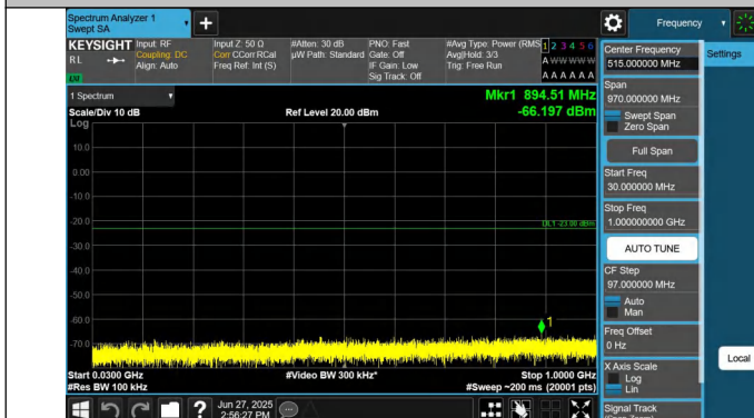
66-66-10MHz-20MHz-QPSK-QPSK-132428-132572-1RB#49-0R B#0-30~1000MHz-PASS
