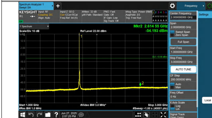
66-66-10MHz-20MHz-QPSK-QPSK-132428-132572-1RB#0-1RB #99-1000~3000MHz-PASS
