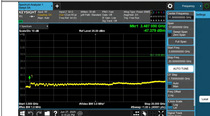
66-66-15MHz-10MHz-QPSK-QPSK-132373-132493-1RB#0-0RB #0-3000~20000MHz-PASS
