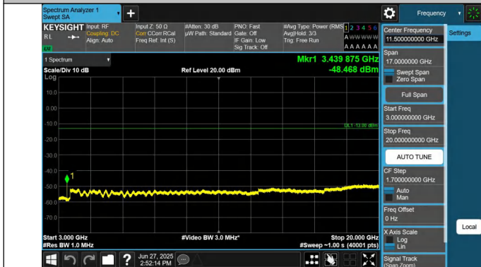
66-66-10MHz-20MHz-QPSK-QPSK-132027-132171-1RB#49-0R B#0-3000~20000MHz-PASS
