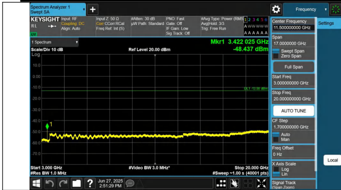
66-66-10MHz-20MHz-QPSK-QPSK-132027-132171-1RB#0-0RB #0-3000~20000MHz-PASS
