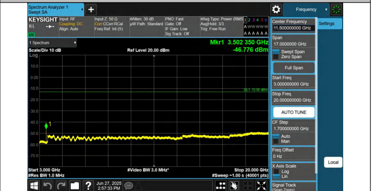
66-66-10MHz-20MHz-QPSK-QPSK-132428-132572-1RB#0-1RB #99-3000~20000MHz-PASS
