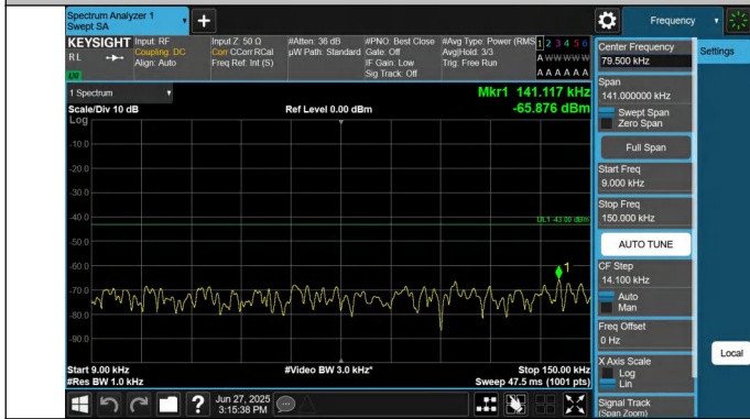
66-66-15MHz-10MHz-QPSK-QPSK-132373-132493-1RB#74-0R B#0-0.009~0.15MHz-PASS
