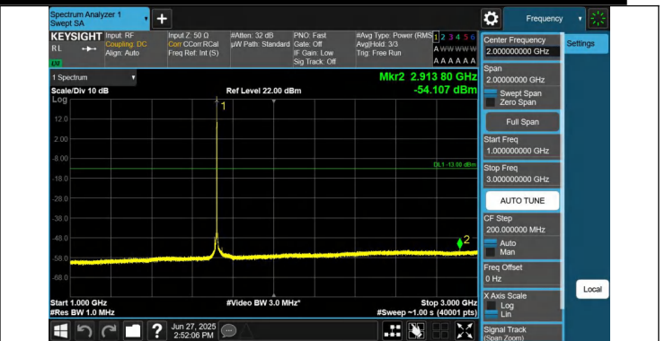
66-66-10MHz-20MHz-QPSK-QPSK-132027-132171-1RB#49-0R B#0-1000~3000MHz-PASS
