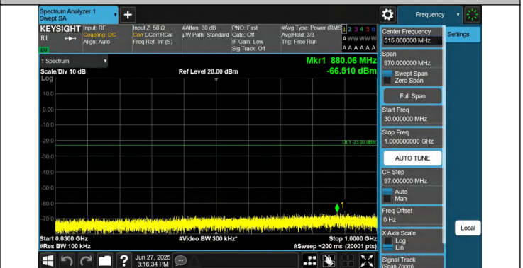
66-66-15MHz-10MHz-QPSK-QPSK-132373-132493-1RB#0-1RB #49-30~1000MHz-PASS
