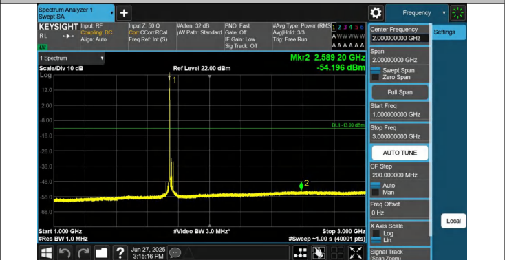
66-66-15MHz-10MHz-QPSK-QPSK-132373-132493-1RB#0-0RB #0-1000~3000MHz-PASS
