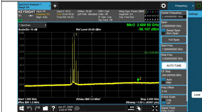
66-66-10MHz-20MHz-QPSK-QPSK-132027-132171-1RB#0-1RB #99-1000~3000MHz-PASS
