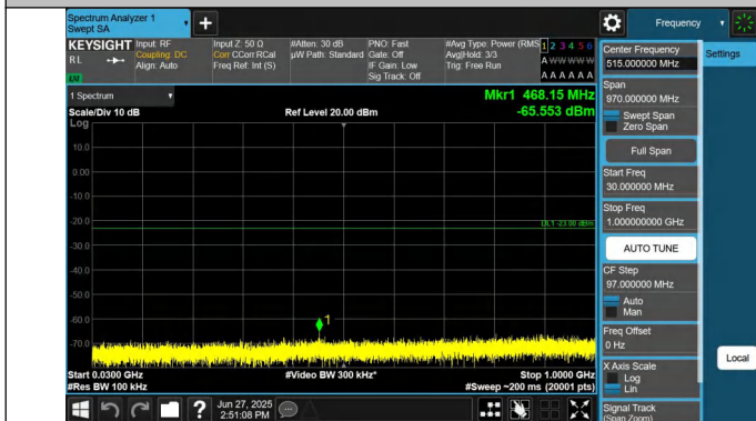
66-66-10MHz-20MHz-QPSK-QPSK-132027-132171-1RB#0-0RB #0-30~1000MHz-PASS
