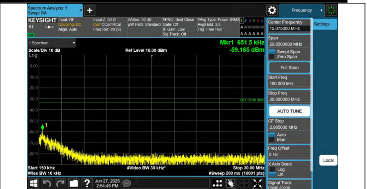
66-66-10MHz-20MHz-QPSK-QPSK-132328-132472-1RB#0-1RB #99-0.15~30MHz-PASS
