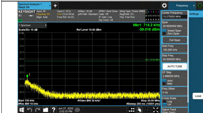
66-66-10MHz-20MHz-QPSK-QPSK-132027-132171-1RB#0-1RB #99-0.15~30MHz-PASS
