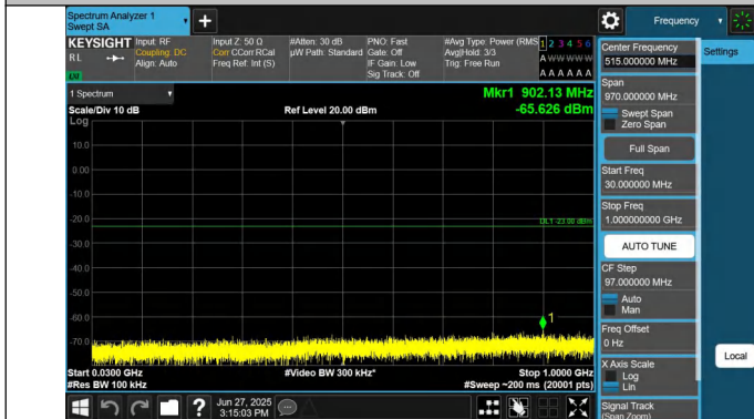
66-66-15MHz-10MHz-QPSK-QPSK-132373-132493-1RB#0-0RB #0-30~1000MHz-PASS
