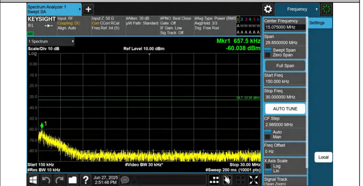
66-66-10MHz-20MHz-QPSK-QPSK-132027-132171-1RB#49-0R B#0-0.15~30MHz-PASS
