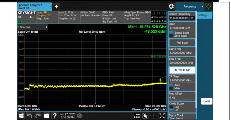
66-66-15MHz-10MHz-QPSK-QPSK-132373-132493-1RB#0-1RB #49-3000~20000MHz-PASS
