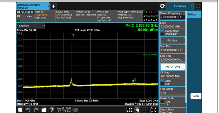
66-66-10MHz-20MHz-QPSK-QPSK-132027-132171-1RB#0-0RB #0-1000~3000MHz-PASS
