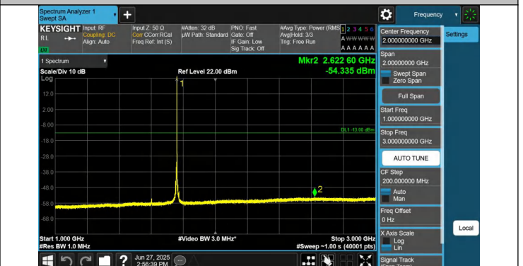
66-66-10MHz-20MHz-QPSK-QPSK-132428-132572-1RB#49-0R B#0-1000~3000MHz-PASS
