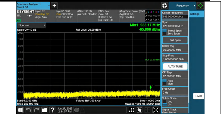
66-66-10MHz-15MHz-QPSK-QPSK-132477-132597-1RB#49-0R B#0-30~1000MHz-PASS
