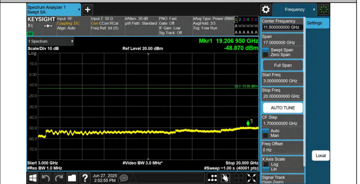
66-66-10MHz-20MHz-QPSK-QPSK-132027-132171-1RB#0-1RB #99-3000~20000MHz-PASS
