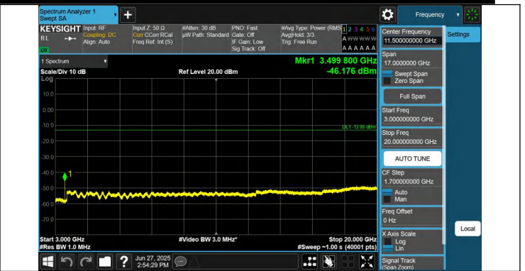
66-66-10MHz-20MHz-QPSK-QPSK-132328-132472-1RB#49-0R B#0-3000~20000MHz-PASS
