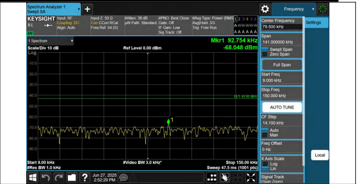
66-66-10MHz-20MHz-QPSK-QPSK-132027-132171-1RB#0-1RB #99-0.009~0.15MHz-PASS
