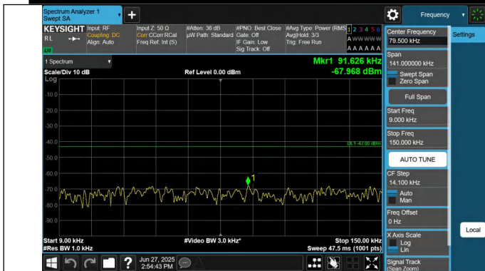
66-66-10MHz-20MHz-QPSK-QPSK-132328-132472-1RB#0-1RB #99-0.009~0.15MHz-PASS
