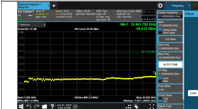
66-66-10MHz-20MHz-QPSK-QPSK-132328-132472-1RB#0-1RB #99-3000~20000MHz-PASS
