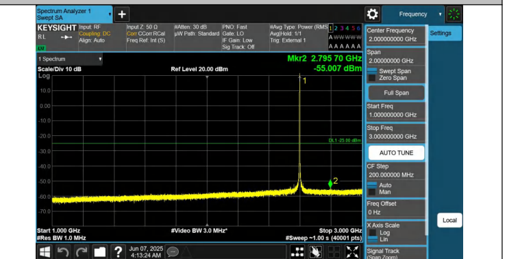
41-41-20MHz-10MHz-QPSK-QPSK-40571-40715-1RB#99-0RB#0 -1000~3000MHz-PASS
