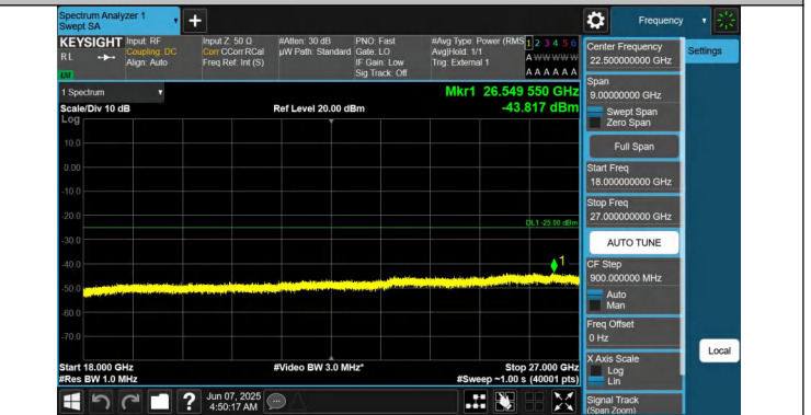
41-41-20MHz-15MHz-QPSK-QPSK-40546-40717-1RB#99-0RB#0 -18000~27000MHz-PASS
