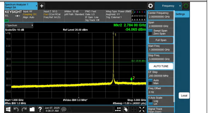
41-41-20MHz-10MHz-QPSK-QPSK-39750-39894-1RB#99-0RB#0 -1000~3000MHz-PASS
