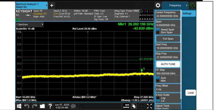
41-41-20MHz-15MHz-QPSK-QPSK-40546-40717-1RB#0-1RB#74 -18000~27000MHz-PASS
