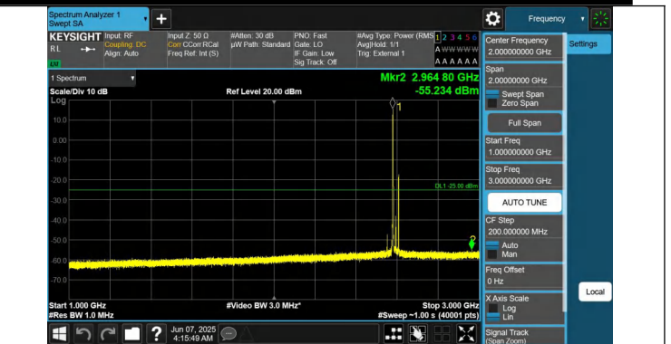
41-41-20MHz-10MHz-QPSK-QPSK-40571-40715-1RB#0-1RB#49 -1000~3000MHz-PASS
