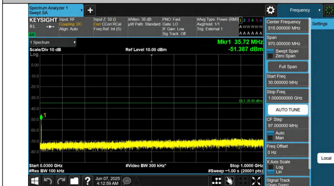
41-41-20MHz-10MHz-QPSK-QPSK-40571-40715-1RB#99-0RB# 0-30~1000MHz-PASS
