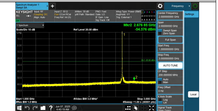
41-41-20MHz-15MHz-QPSK-QPSK-39750-39921-1RB#0-0RB#0- 1000~3000MHz-PASS
