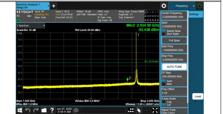
41-41-20MHz-10MHz-QPSK-QPSK-41391-41535-1RB#0-0RB#0- 1000~3000MHz-PASS
