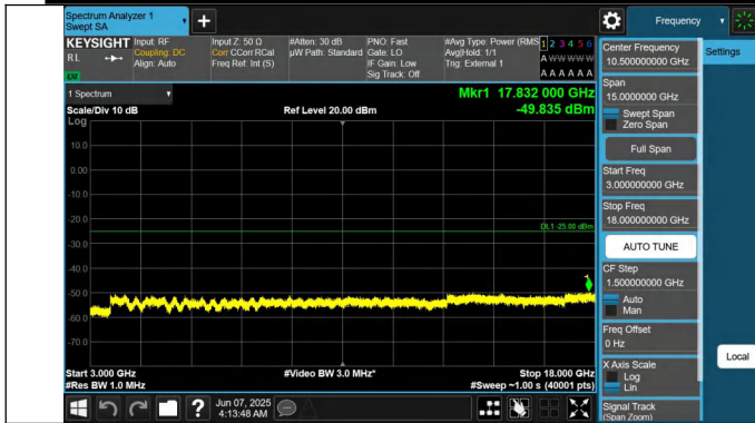
41-41-20MHz-10MHz-QPSK-QPSK-40571-40715-1RB#99-0RB# 0-3000~18000MHz-PASS
