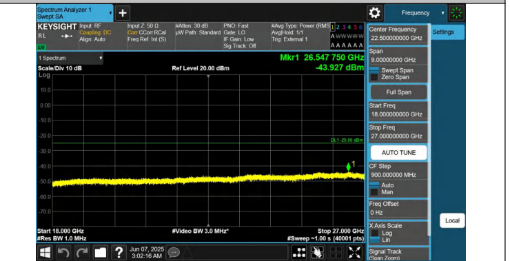
41-41-15MHz-20MHz-QPSK-QPSK-40523-40694-75RB#0-100RB #0-18000~27000MHz-PASS
