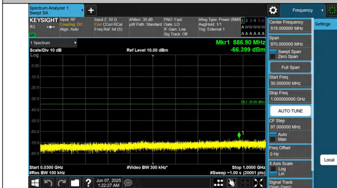
41-41-10MHz-20MHz-QPSK-QPSK-39705-39849-1RB#0-1RB#99-9-30~1000MHz-PASS
