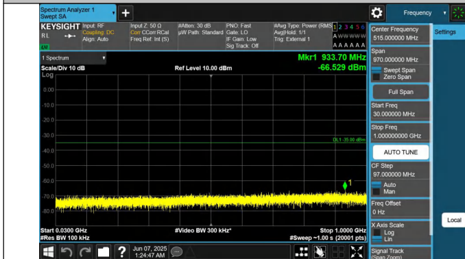
41-41-10MHz-20MHz-QPSK-QPSK-40526-40670-1RB#0-0RB#0- 30~1000MHz-PASS
