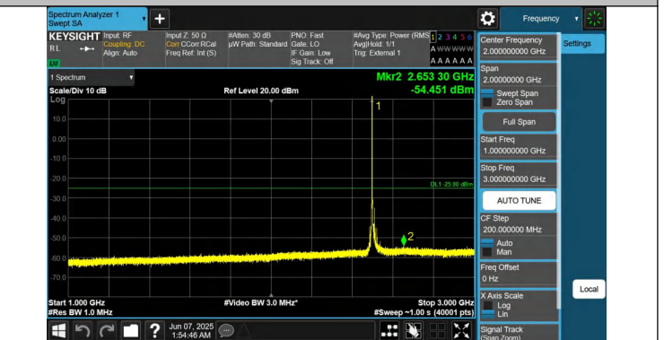
41-41-15MHz-10MHz-QPSK-QPSK-39725-39845-1RB#0-0RB#0- 1000~3000MHz-PASS
