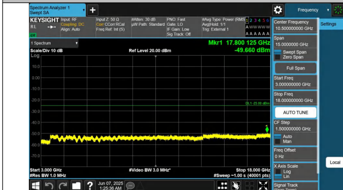
41-41-10MHz-20MHz-QPSK-QPSK-40526-40670-1RB#0-0RB#0- 3000~18000MHz-PASS
