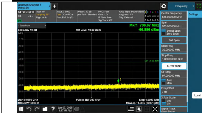
41-41-10MHz-20MHz-QPSK-QPSK-39705-39849-1RB#0-0RB#0-30~1000MHz-PASS
