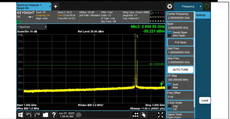
41-41-10MHz-20MHz-QPSK-QPSK-40526-40670-1RB#0-1RB#99 -1000~3000MHz-PASS
