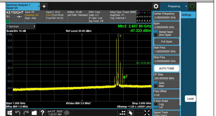
41-41-10MHz-20MHz-QPSK-QPSK-39705-39849-1RB#0-1RB#99-1000~3000MHz-PASS
