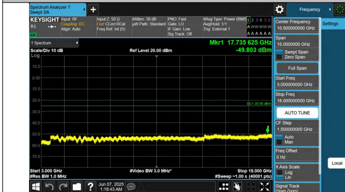
41-41-10MHz-20MHz-QPSK-QPSK-39705-39849-1RB#0-0RB#0-3000~18000MHz-PASS
