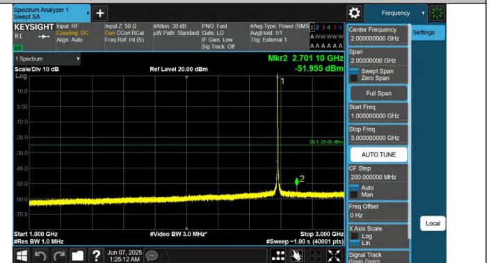
41-41-10MHz-20MHz-QPSK-QPSK-40526-40670-1RB#0-0RB#0- 1000~3000MHz-PASS
