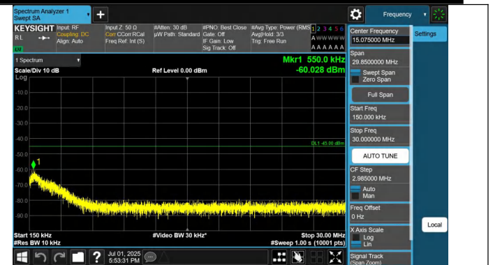
41-41-10MHz-20MHz-QPSK-QPSK-40526-40670-1RB#0-0RB#0- 0.15~30MHz-PASS
