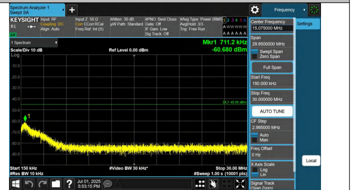
41-41-10MHz-20MHz-QPSK-QPSK-39705-39849-1RB#0-1RB#99-0.15~30MHz-PASS
