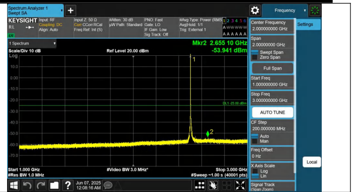
41-41-5MHz-20MHz-QPSK-QPSK-39683-39800-1RB#24-0RB#0-1000~3000MHz-PASS
