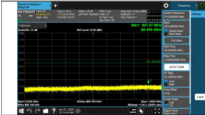
41-41-5MHz-20MHz-QPSK-QPSK-40528-40645-1RB#24-0RB#0- 30~1000MHz-PASS
