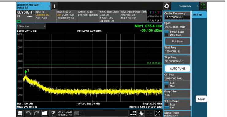
41-41-5MHz-20MHz-QPSK-QPSK-41373-41490-1RB#0-1RB#99- 0.15~30MHz-PASS
