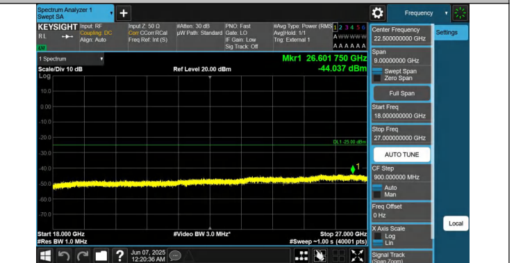
41-41-5MHz-20MHz-QPSK-QPSK-41373-41490-1RB#0-0RB#0-1 8000~27000MHz-PASS
