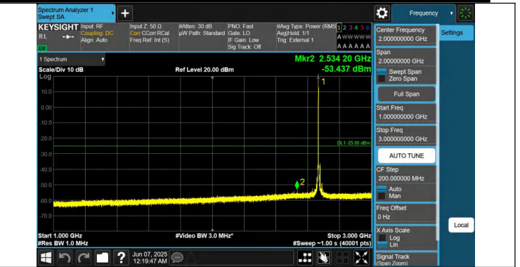
41-41-5MHz-20MHz-QPSK-QPSK-41373-41490-1RB#0-0RB#0-1 000~3000MHz-PASS
