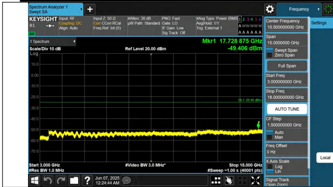
41-41-5MHz-20MHz-QPSK-QPSK-41373-41490-1RB#0-1RB#99- 3000~18000MHz-PASS
