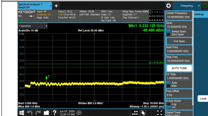
41-41-5MHz-20MHz-QPSK-QPSK-41373-41490-1RB#0-0RB#0-3 000~18000MHz-PASS
