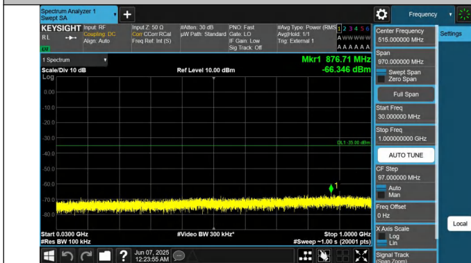
41-41-5MHz-20MHz-QPSK-QPSK-41373-41490-1RB#0-1RB#99- 30~1000MHz-PASS
