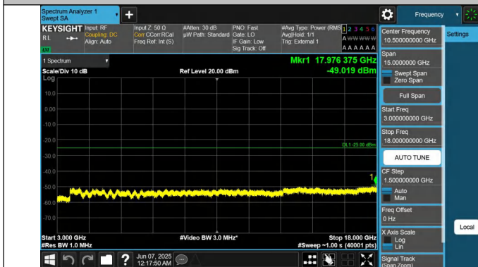
41-41-5MHz-20MHz-QPSK-QPSK-40528-40645-1RB#0-1RB#99- 3000~18000MHz-PASS
