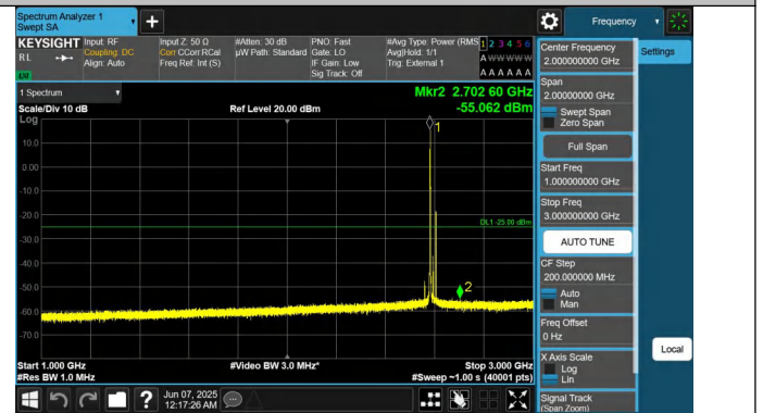
41-41-5MHz-20MHz-QPSK-QPSK-40528-40645-1RB#0-1RB#99- 1000~3000MHz-PASS
