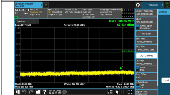
41-41-5MHz-20MHz-QPSK-QPSK-40528-40645-1RB#0-1RB#99- 30~1000MHz-PASS
