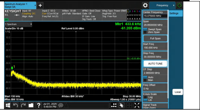
41-41-5MHz-20MHz-QPSK-QPSK-40528-40645-1RB#24-0RB#0- 0.15~30MHz-PASS
