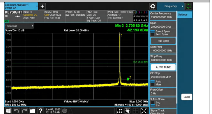
41-41-5MHz-20MHz-QPSK-QPSK-40528-40645-1RB#0-0RB#0-1000~3000MHz-PASS
