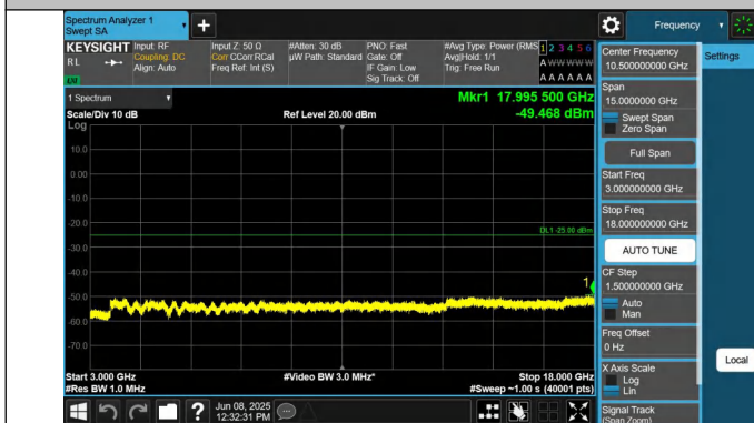
7-7-20MHz-10MHz-QPSK-QPSK-21251-21395-1RB#99-0RB#0- 3000~18000MHz-PASS
