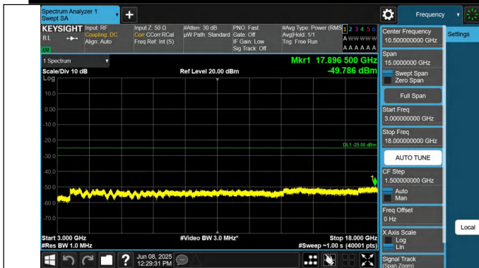
7-7-20MHz-10MHz-QPSK-QPSK-21051-21195-1RB#0-0RB#0-30 00~18000MHz-PASS
