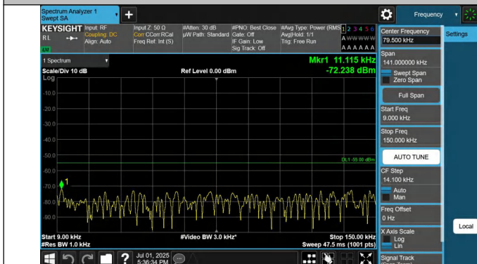
7-7-20MHz-10MHz-QPSK-QPSK-20850-20994-1RB#99-0RB#0-0.009~0.15MHz-PASS
