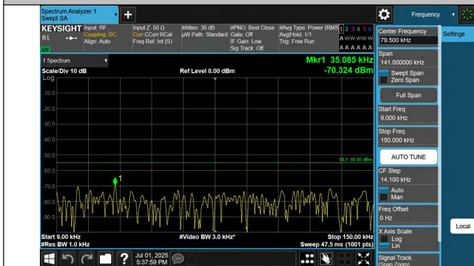
7-7-20MHz-10MHz-QPSK-QPSK-21251-21395-1RB#99-0RB#0- 0.009~0.15MHz-PASS
