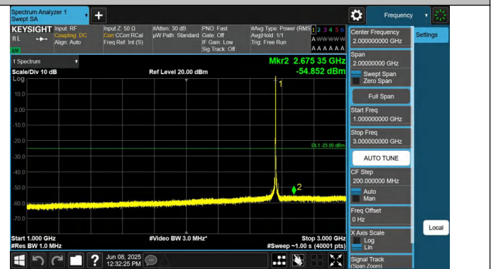
7-7-20MHz-10MHz-QPSK-QPSK-21251-21395-1RB#99-0RB#0-1 000~3000MHz-PASS
