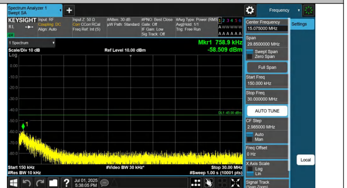
7-7-20MHz-10MHz-QPSK-QPSK-21251-21395-1RB#99-0RB#0-0. 15~30MHz-PASS
