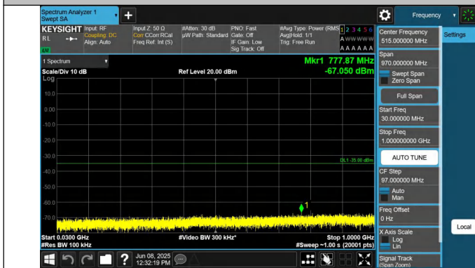
7-7-20MHz-10MHz-QPSK-QPSK-21251-21395-1RB#99-0RB#0- 30~1000MHz-PASS
