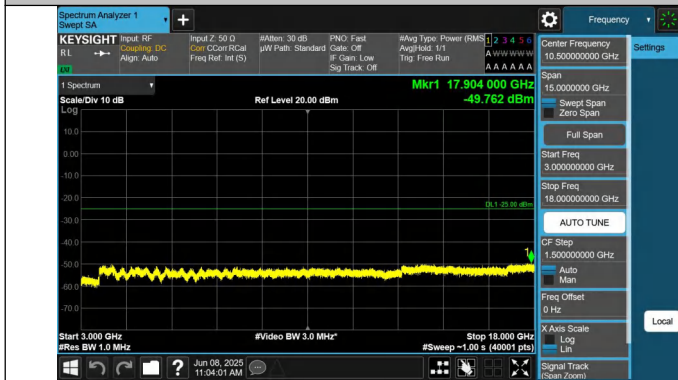
7-7-10MHz-20MHz-QPSK-QPSK-20805-20949-1RB#0-1RB#99- 3000~18000MHz-PASS
