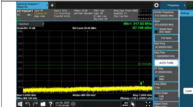
7-7-10MHz-20MHz-QPSK-QPSK-20805-20949-1RB#0-1RB#99- 30~1000MHz-PASS
