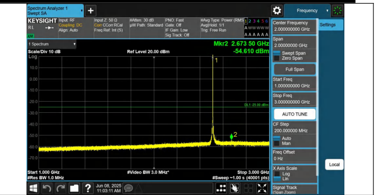
7-7-10MHz-20MHz-QPSK-QPSK-20805-20949-1RB#49-0RB#0-1000~3000MHz-PASS
