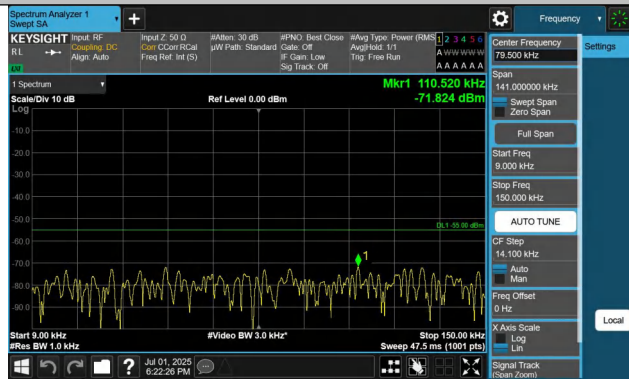
7-7-10MHz-20MHz-QPSK-QPSK-21206-21350-1RB#0-0RB#0-0. 009~0.15MHz-PASS
