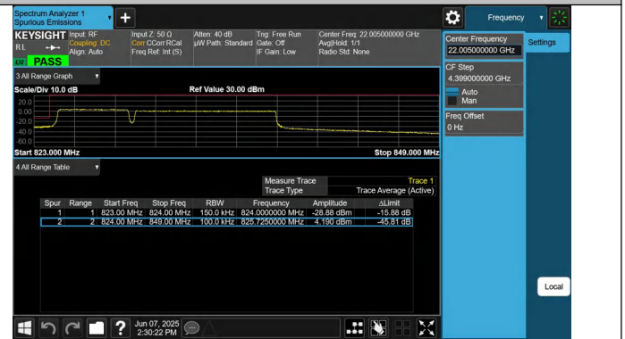
5-5-5MHz-10MHz-QPSK@QPSK-QPSK@QPSK-20428-20500-25 RB#0@25RB#0-50RB#0@50RB#0-PASS
