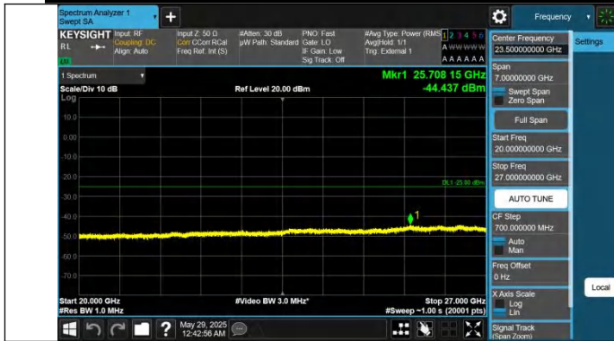
Band41-5MHz-QPSK-41565-1RB#0-20000~27000-PASS
