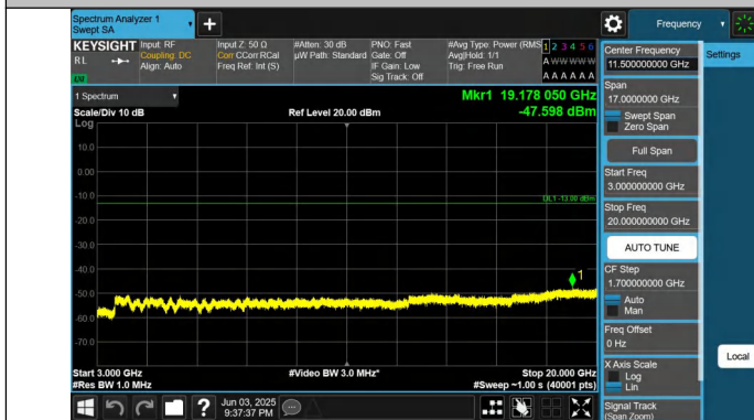
Band25-15MHz-QPSK-26115-1RB#0-3000~20000-PASS
