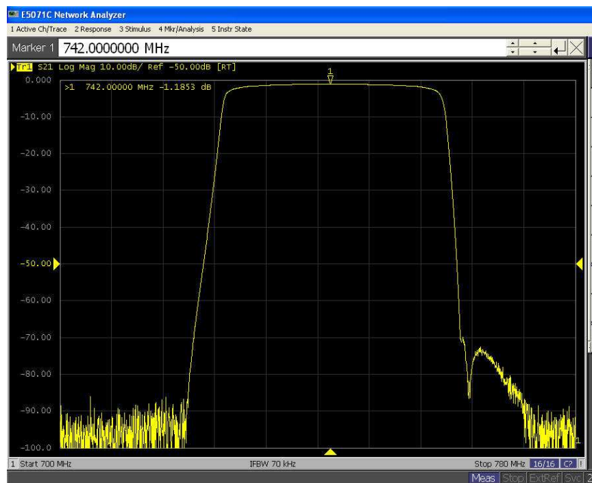
Up-link
