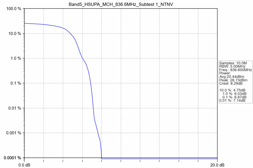
Band5_HSUPA_MCH_836.6MHz_Subtest 1_NTNV
