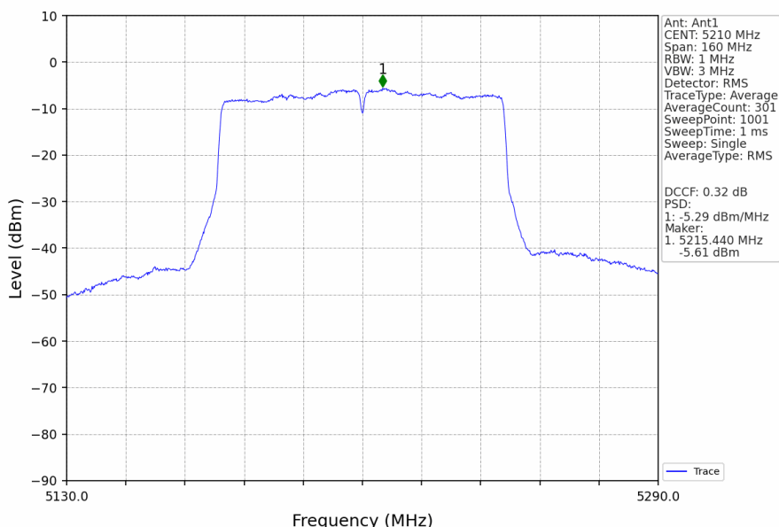
802.11ac(VHT80)_MCH_5210MHz_Ant1_NTNV
