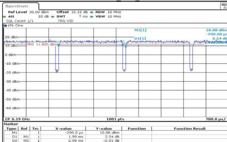
11N40MIMO_Ant1_5190
