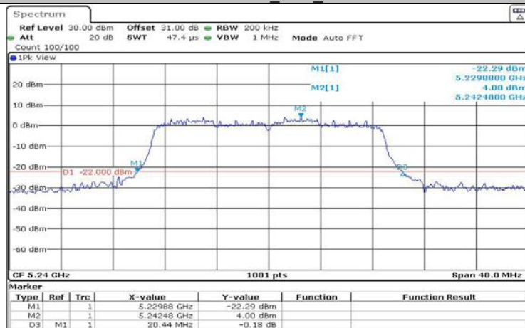
11N20MIMO_Ant1_5240
