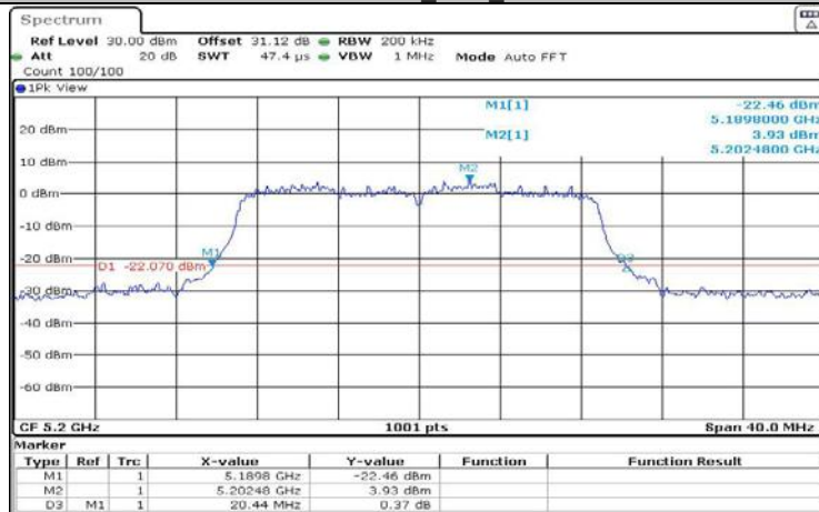
11N20MIMO_Ant1_5200
