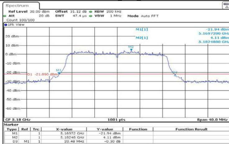
11N20MIMO_Ant1_5180
